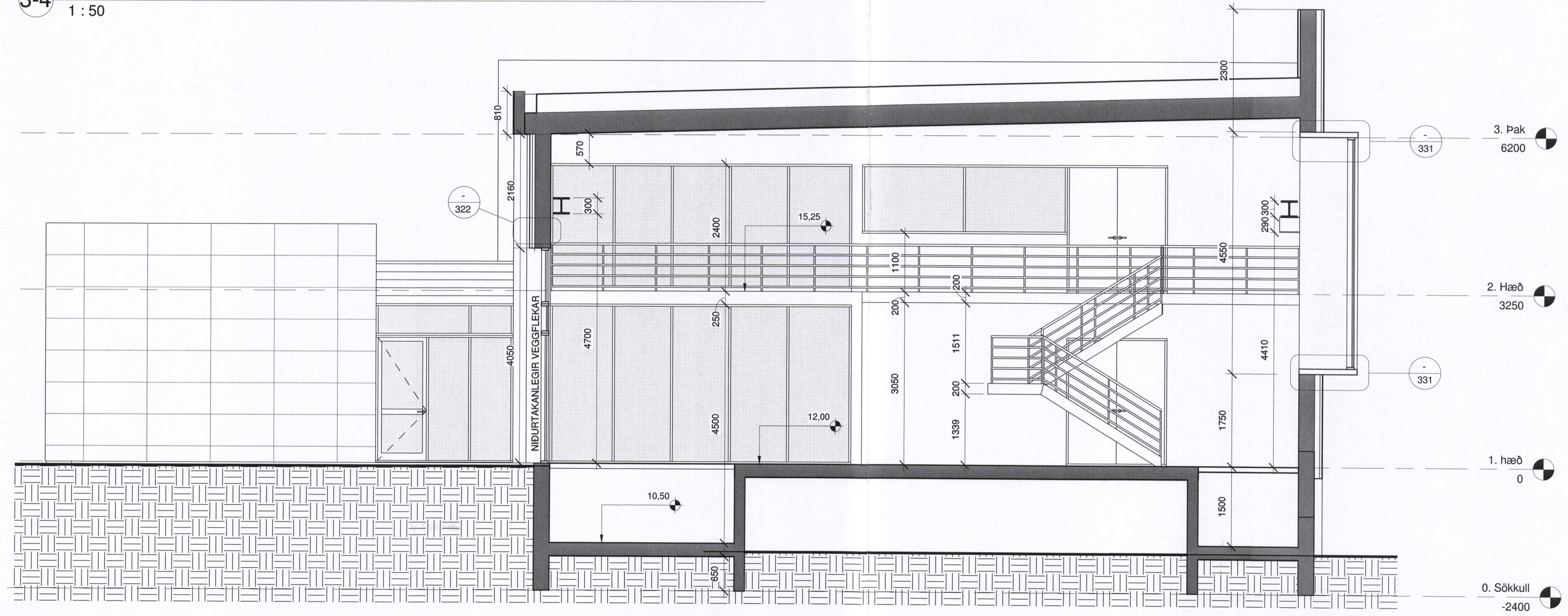
7-6 ÞVERSNIÐ 7-6 1 : 50
