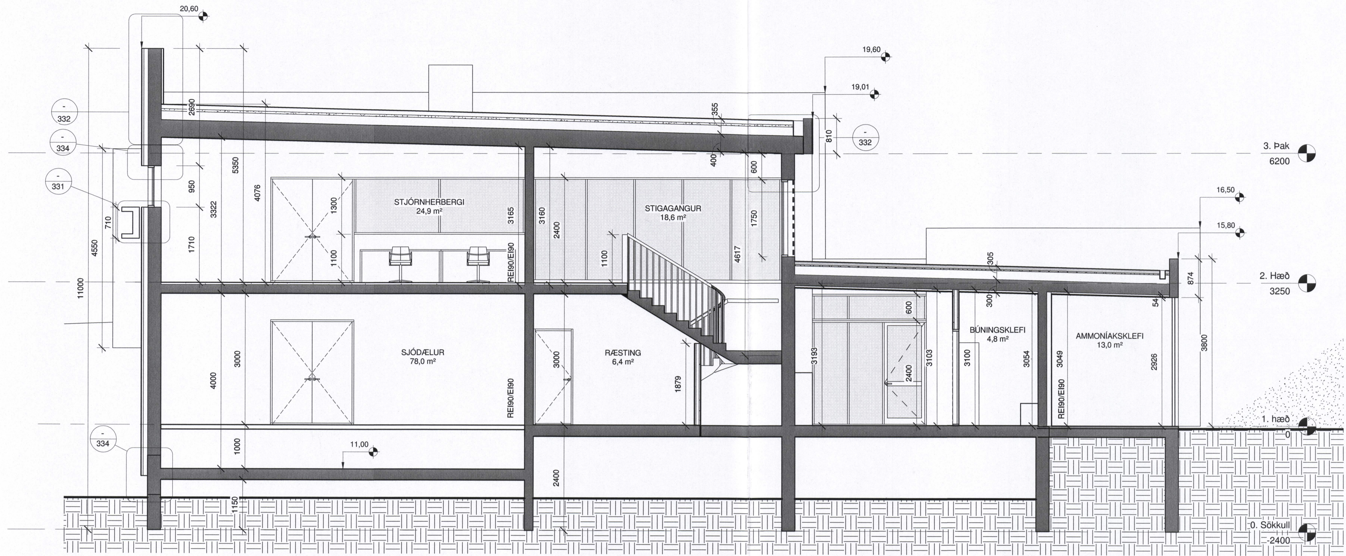
3-4 ÞVERSNIÐ 3-4 1 : 50
