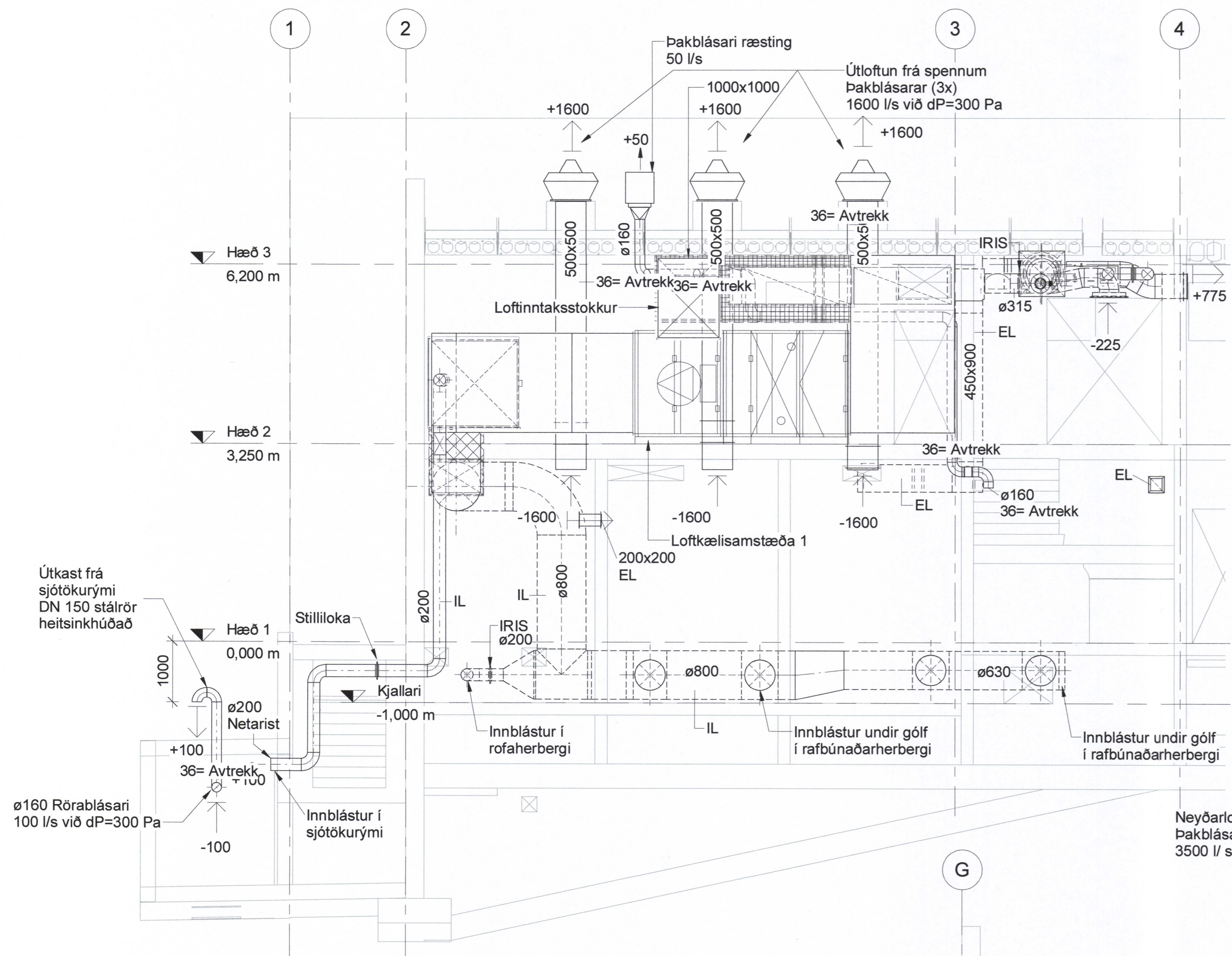
A SNID M47.101 1 : 50
