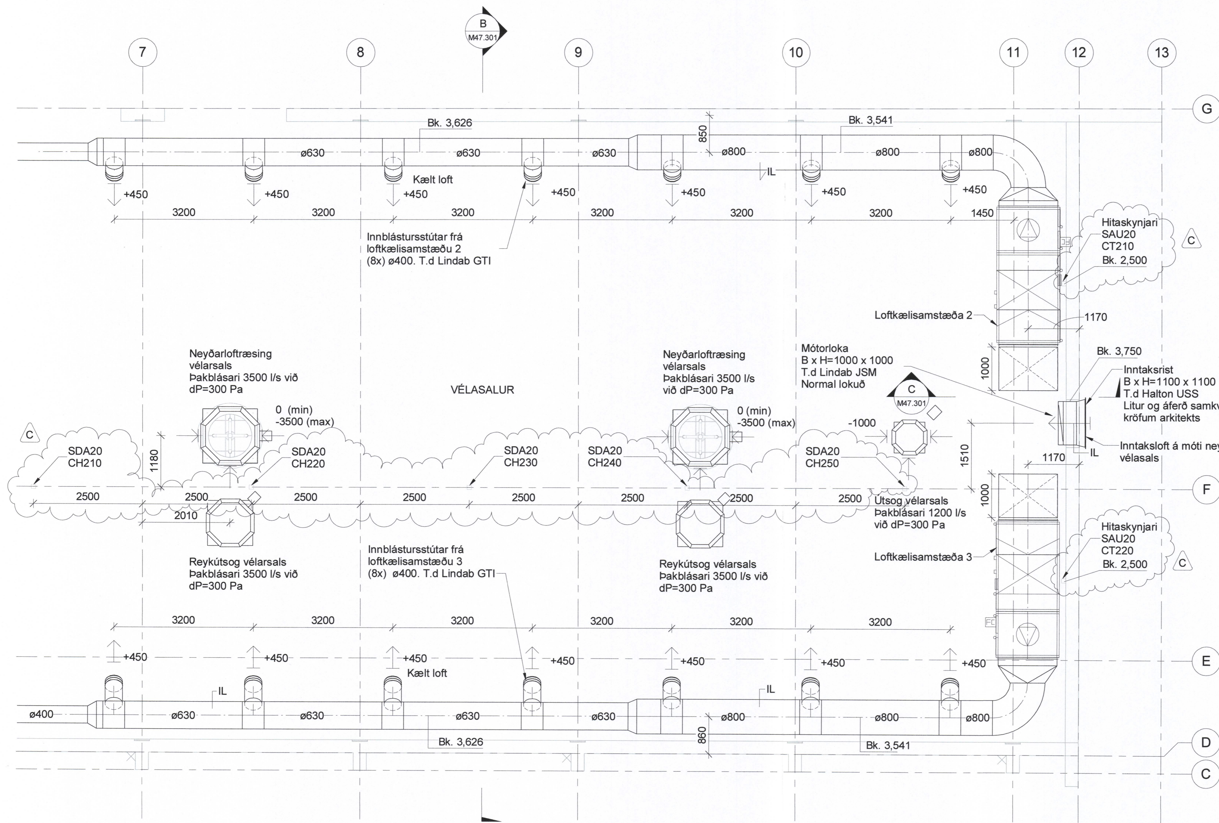
GRUNNMYND 2. HÆÐ 2/2 1 : 50
