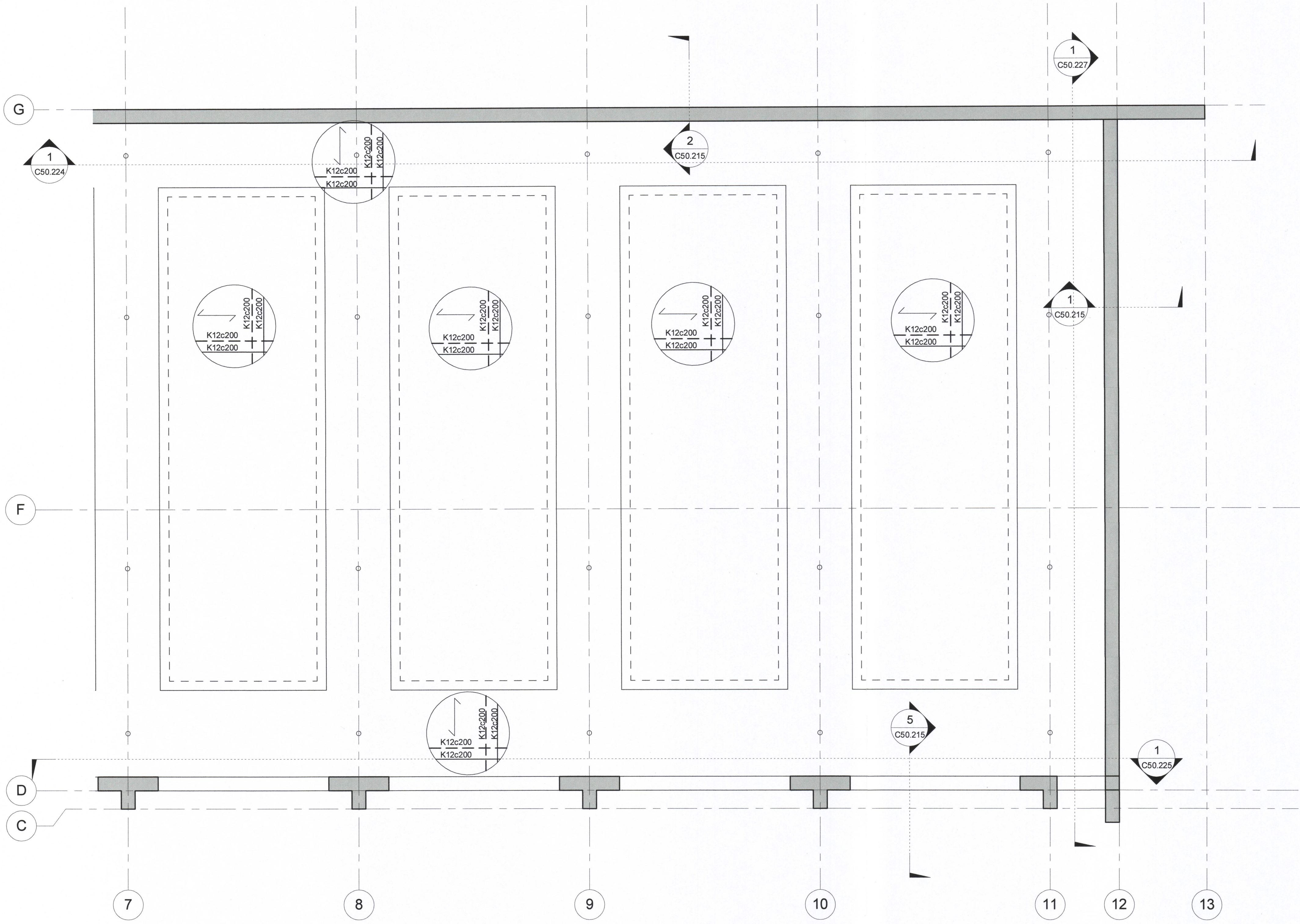
1. hæð Jármateikning 2/2 1 : 50
