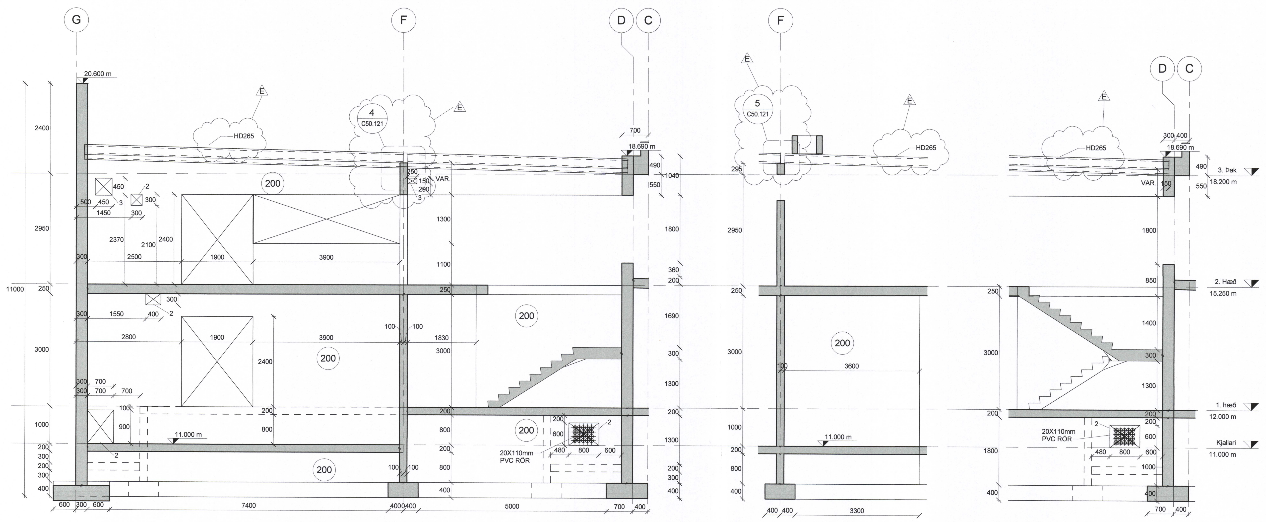
1 SNID C50.101 1 : 50
