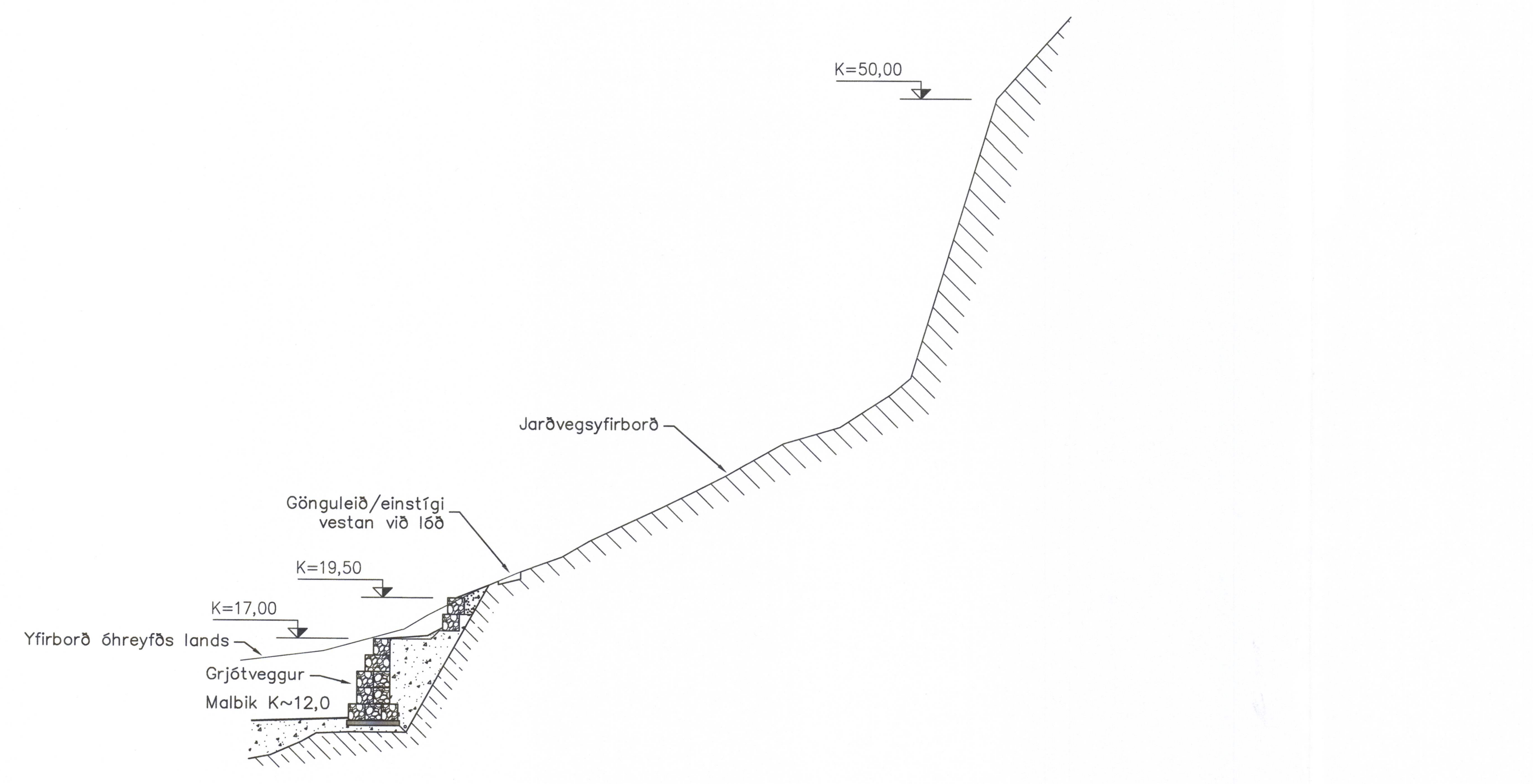
A Þversnið – Grjótveggur og fjallshlíð vestan við lóð (Flatir) 001 1:200
