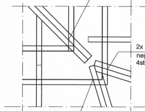
DEILI- C 1:20
