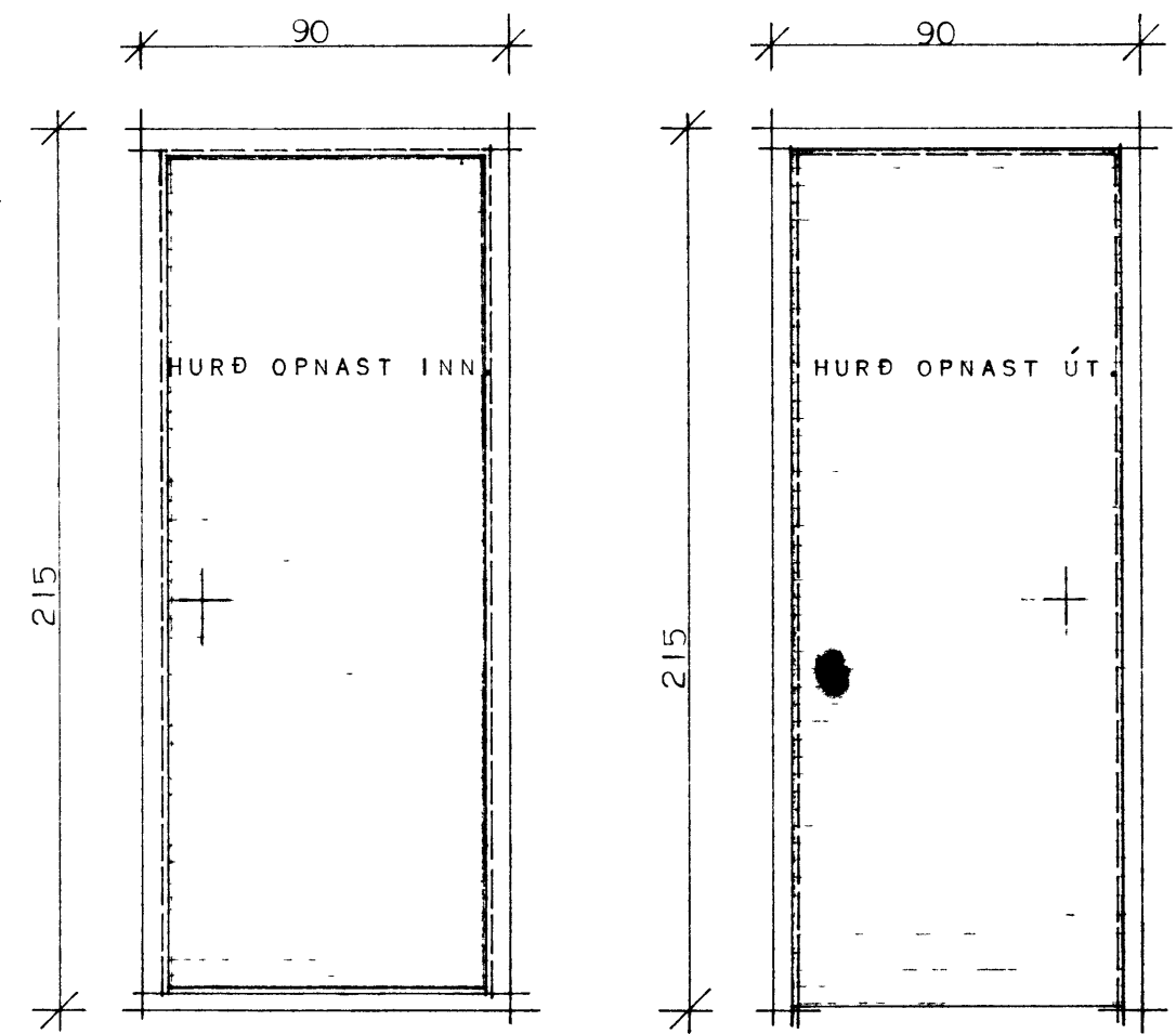
1 STK. Í BÍLGEYMSLU
