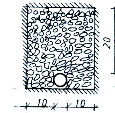
JARÐVATNSLÖGN ÞVERSNÍÐ 1:10
