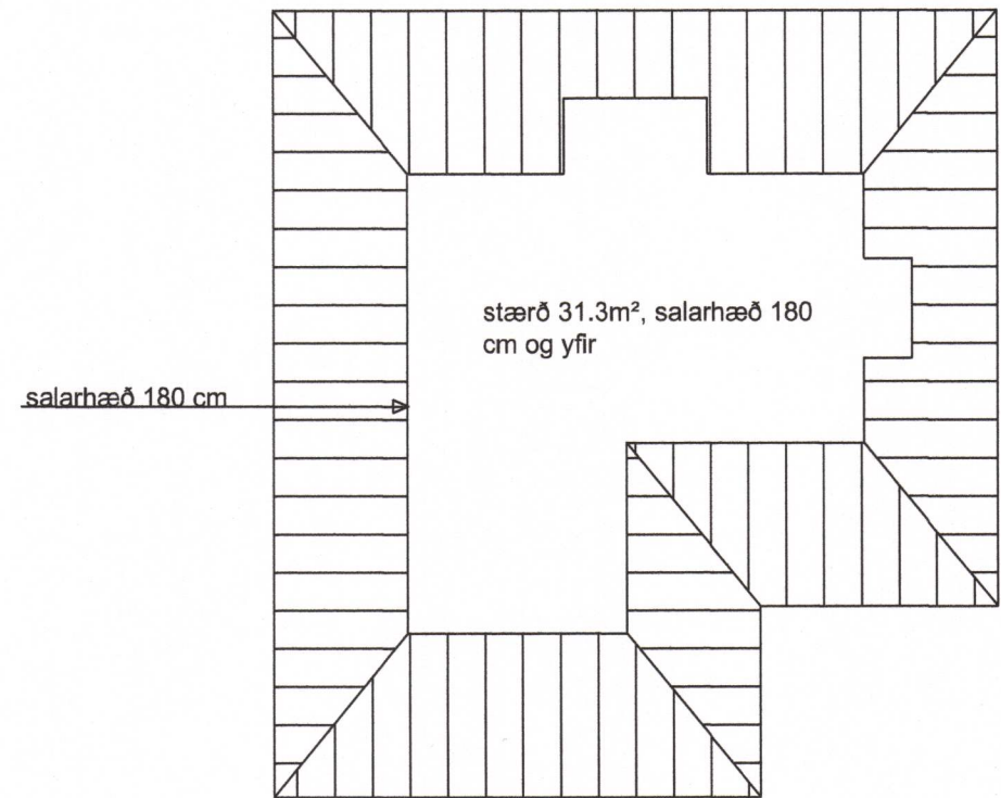
Grunnmynd 3.hæð, mkv 1:100
