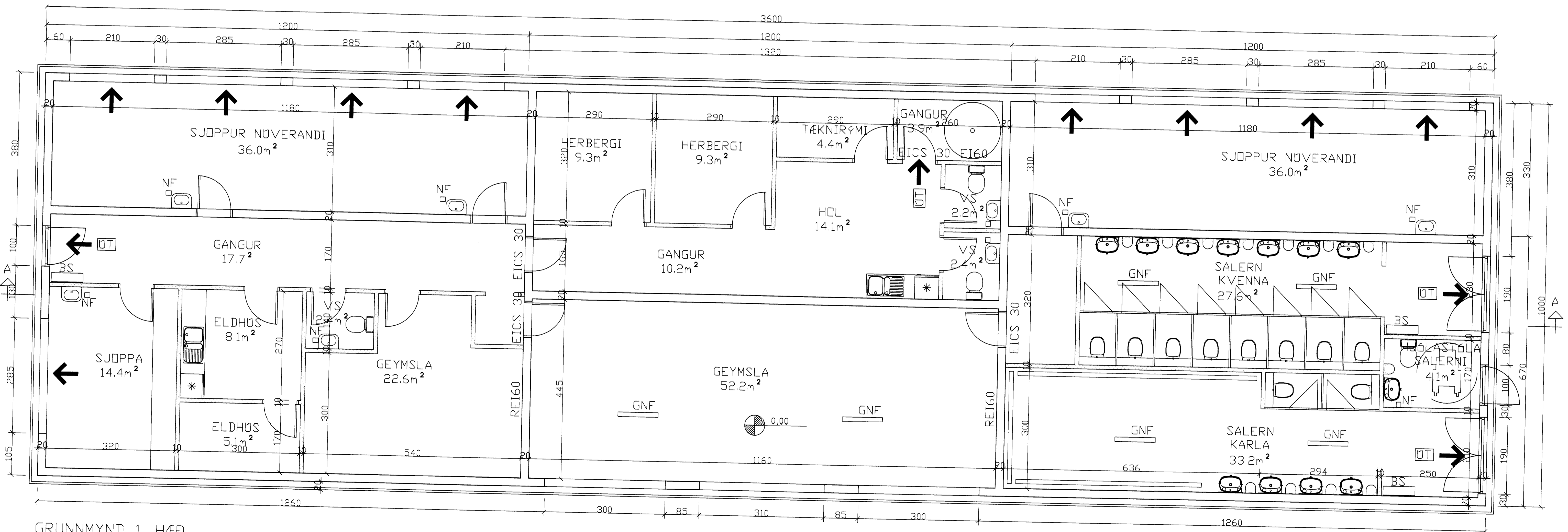
GRUNNMYND 1. HÆÐ
