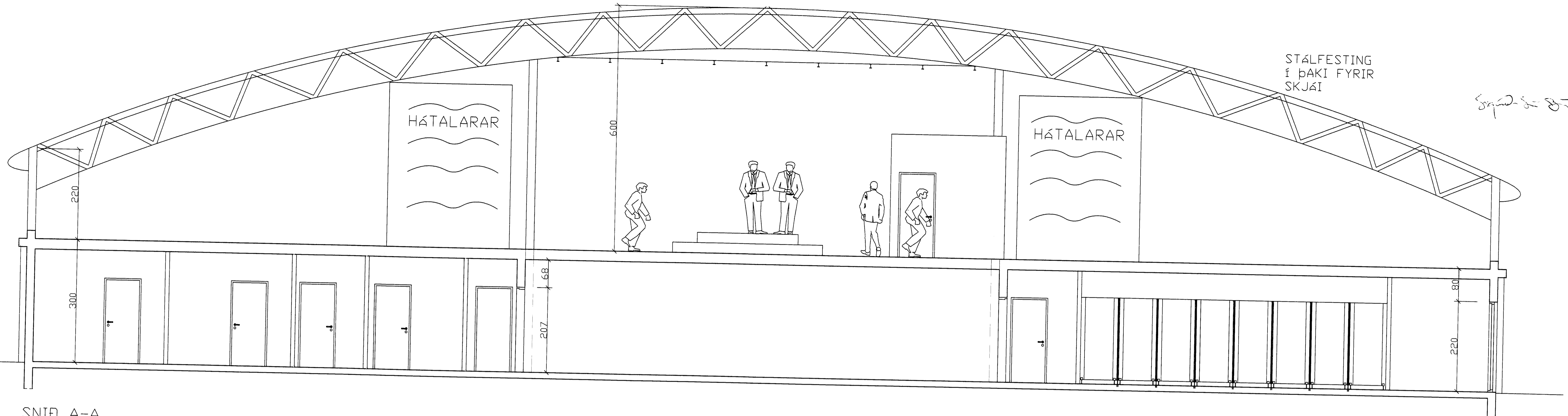
SNIÐ A-A
