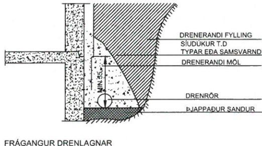
FRÁGANGUR DRENLAGNAR
