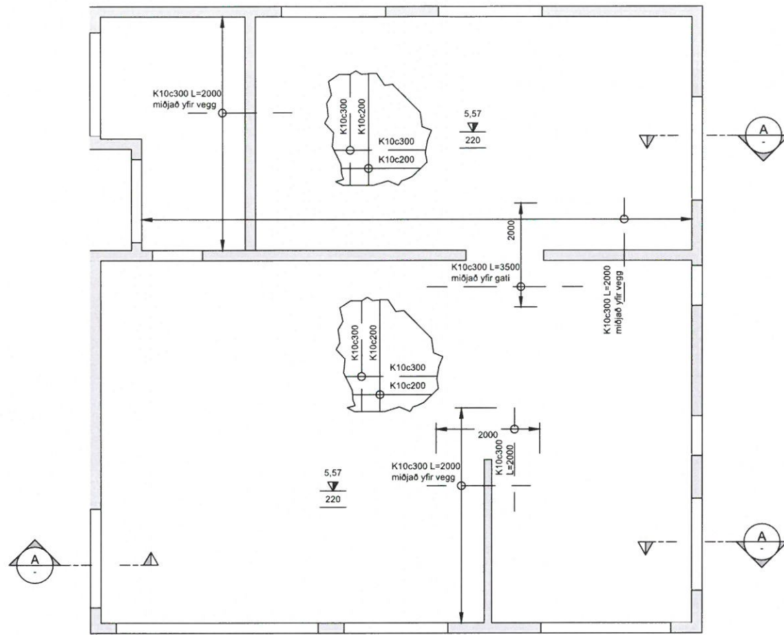
GRUNNMYND, VEGGIR OG LOFTAPLATA 2. HÆÐAR 1:50
