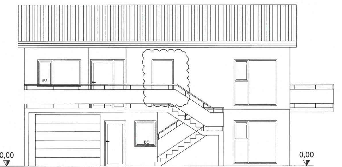
ÚTLIT VESTUR 1:50
