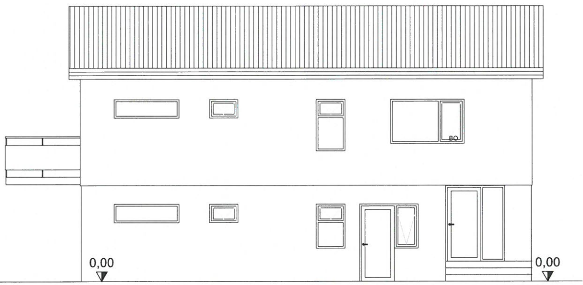
ÚTLIT AUSTUR 1:50
