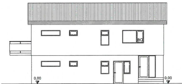
ÚTLIT AUSTUR
