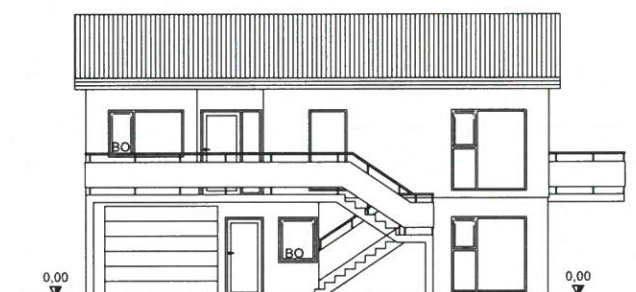
ÚTLIT VESTUR
