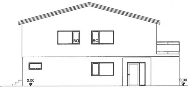
ÚTLIT NORÐUR
