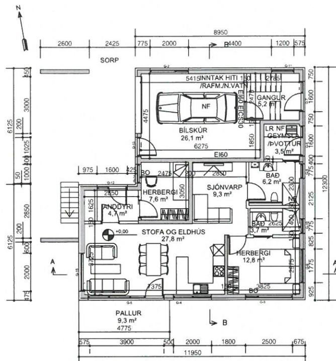
NEDRI HÆÐ, GRUNNMYND
