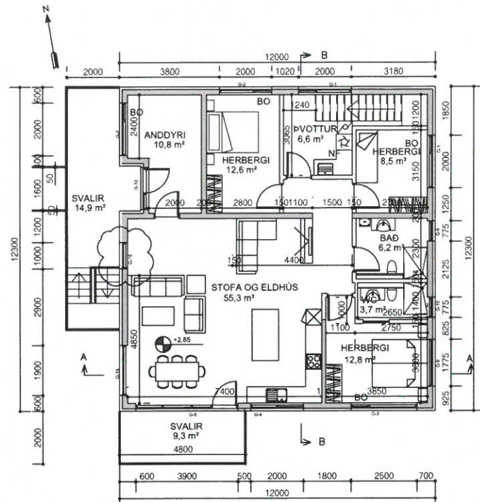
EFRI HÆÐ, GRUNNMYND
