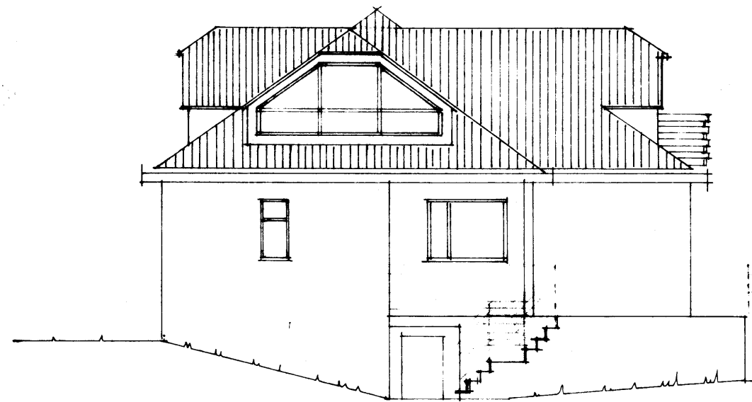
NORÐURHLIÐ
