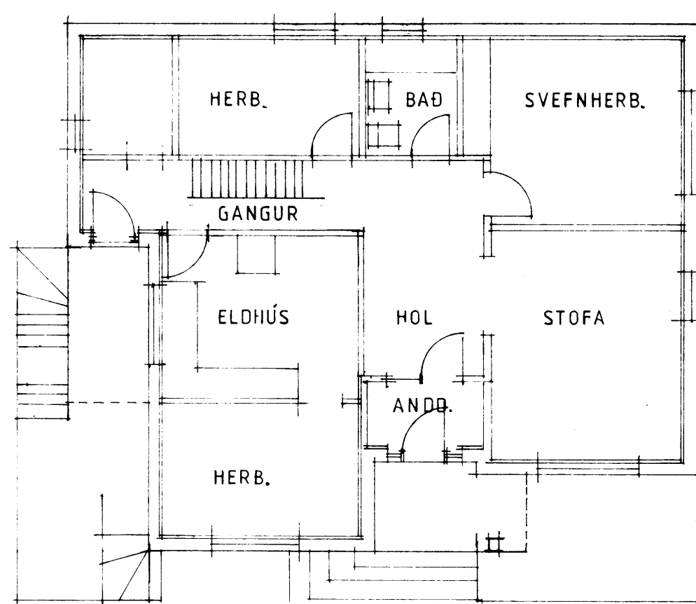
GRUNNMYND 1 HÆÐ 1:100
