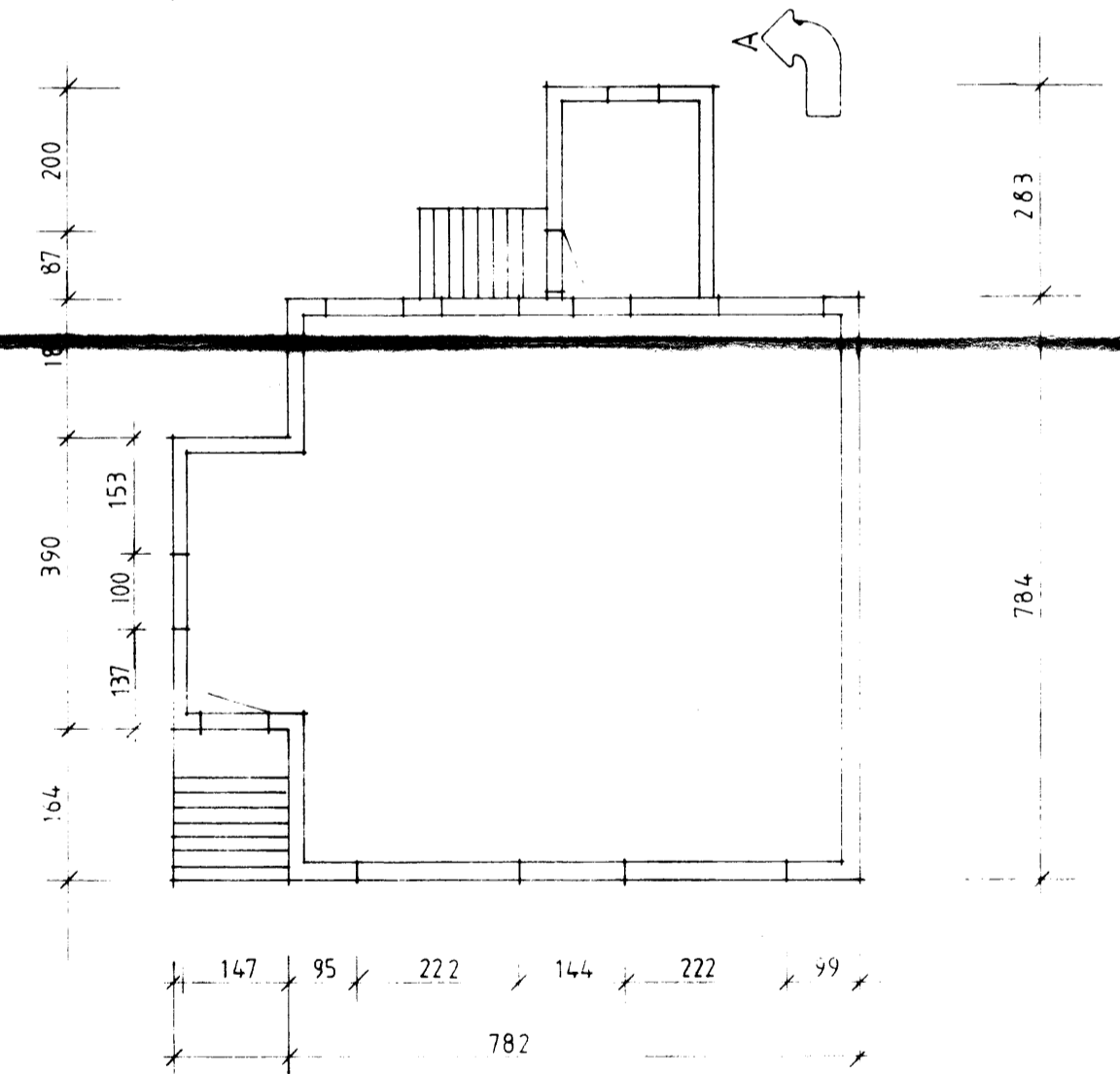
GRUNNMYND 1. HAED
