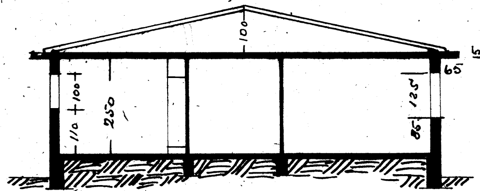
SKURÐUR
