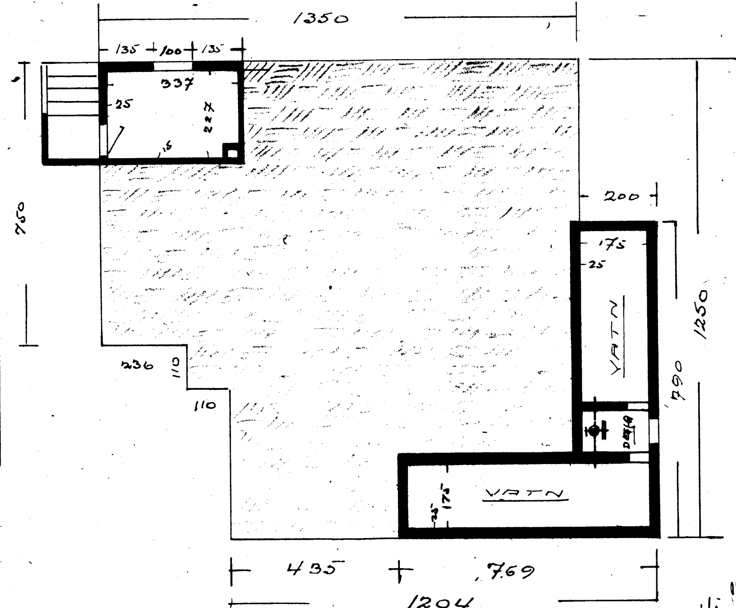
GRUNNFLÖTUR
