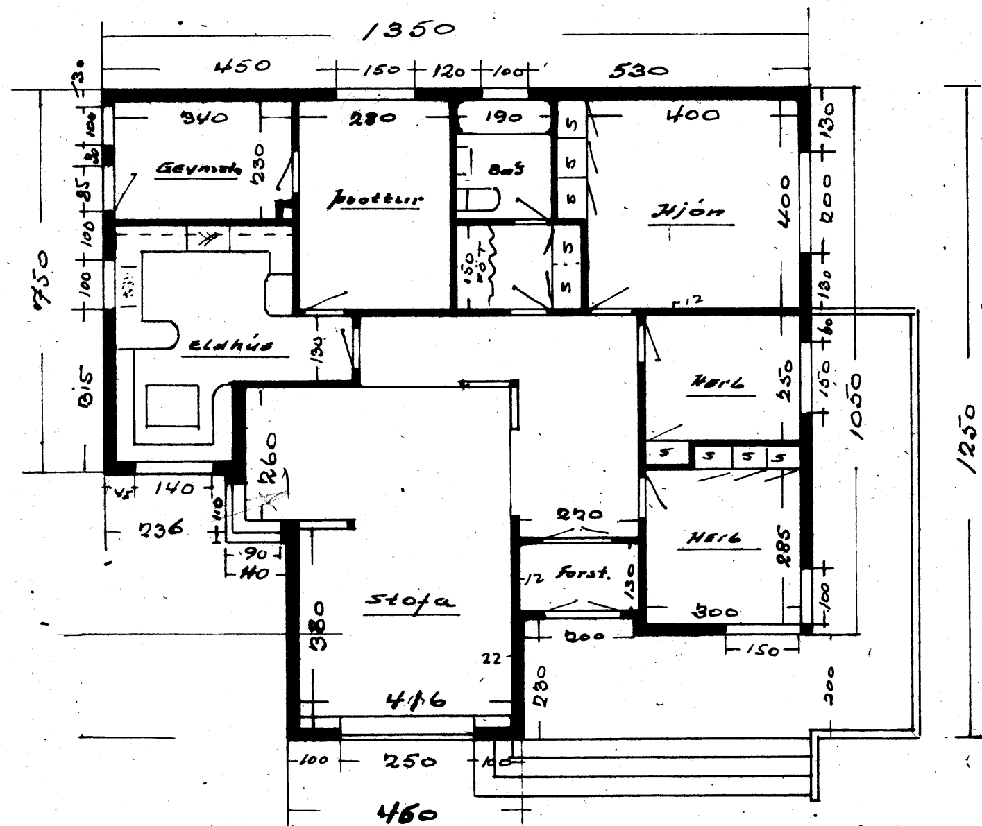
VESTUR
