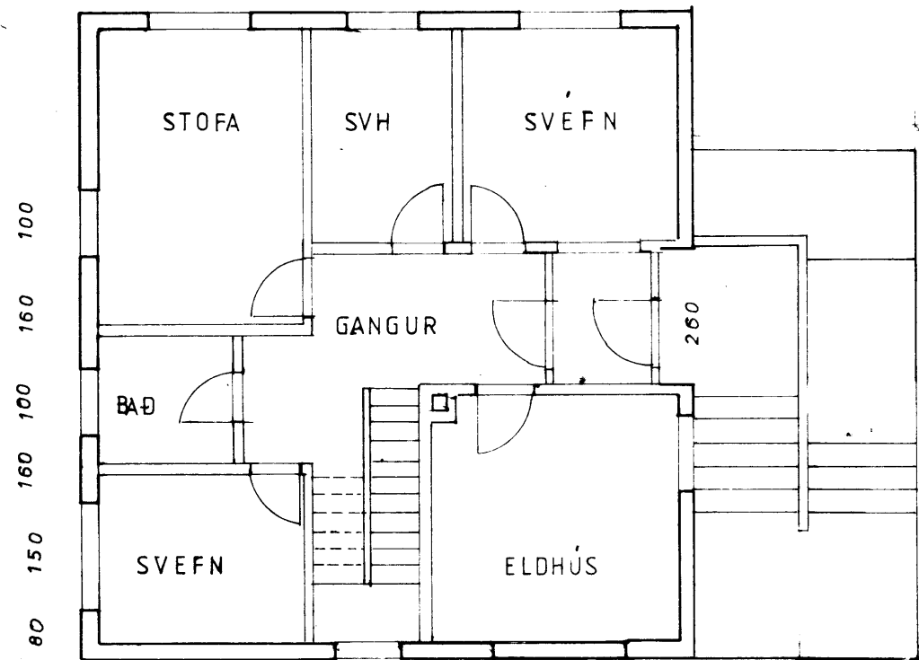
GRUNNMYND 1:100
