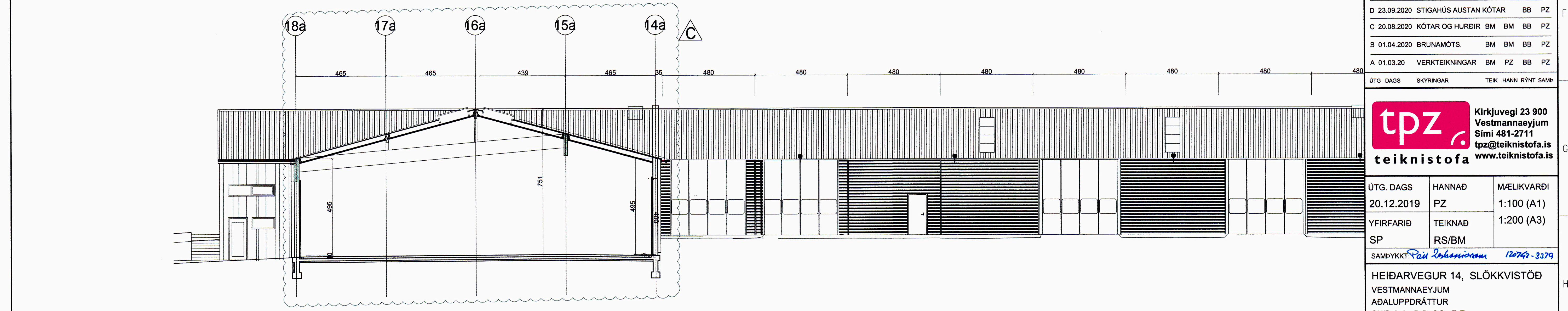
SNID B-B 1:100
