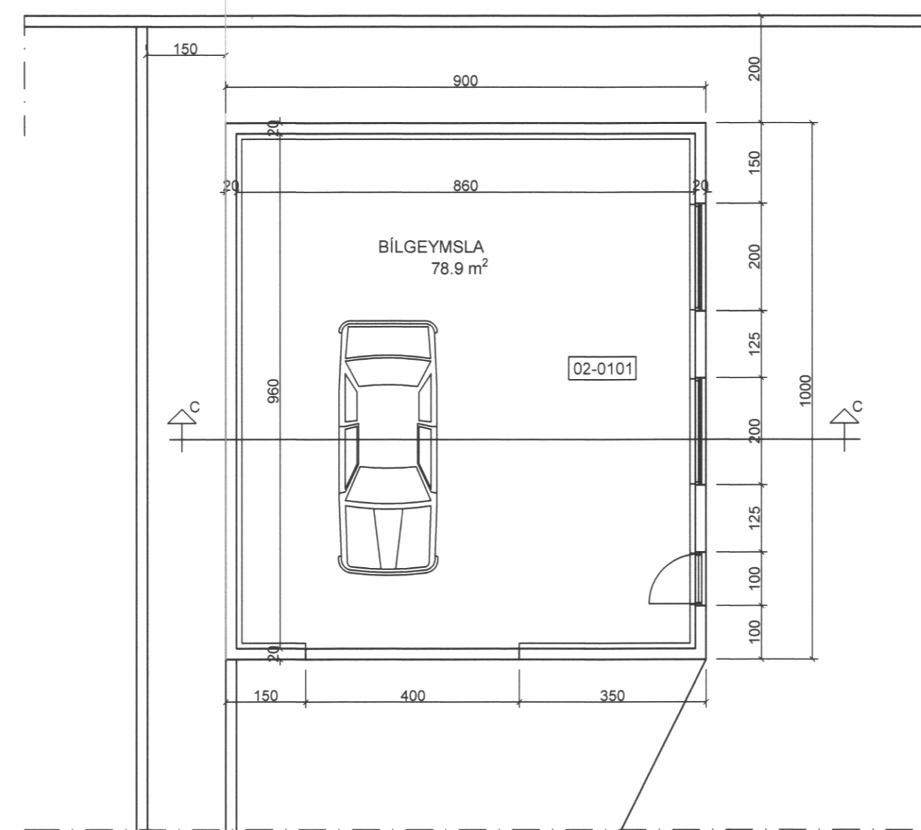
GRUNNMYND BÍLSKÚR 1:100
