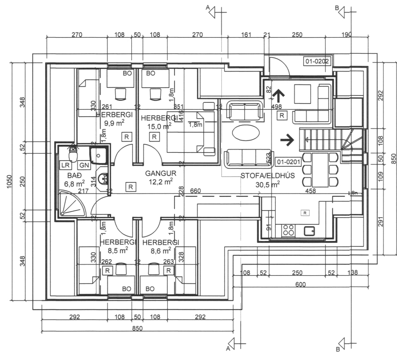
GRUNNMYND RIS 1:100
