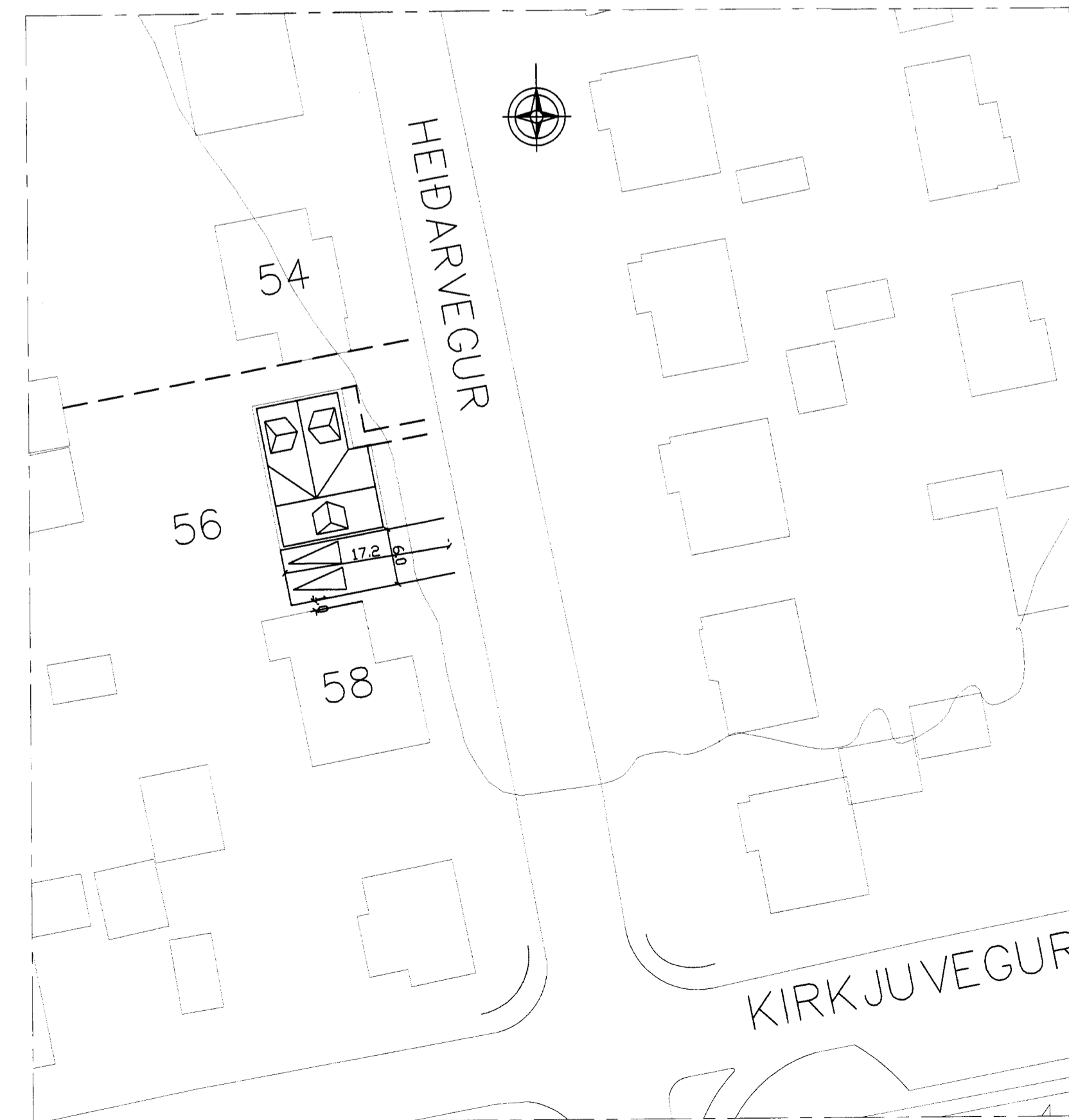
AFSTÖÐUMYND 1:500
