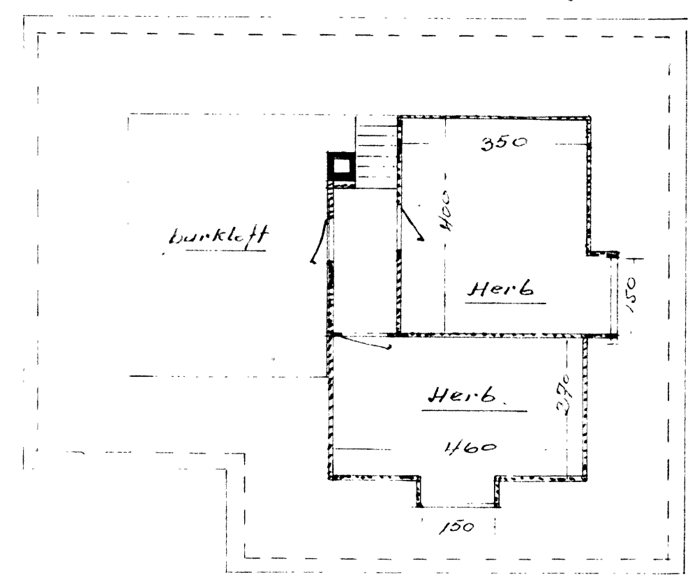
ÞAKHÆÐ
