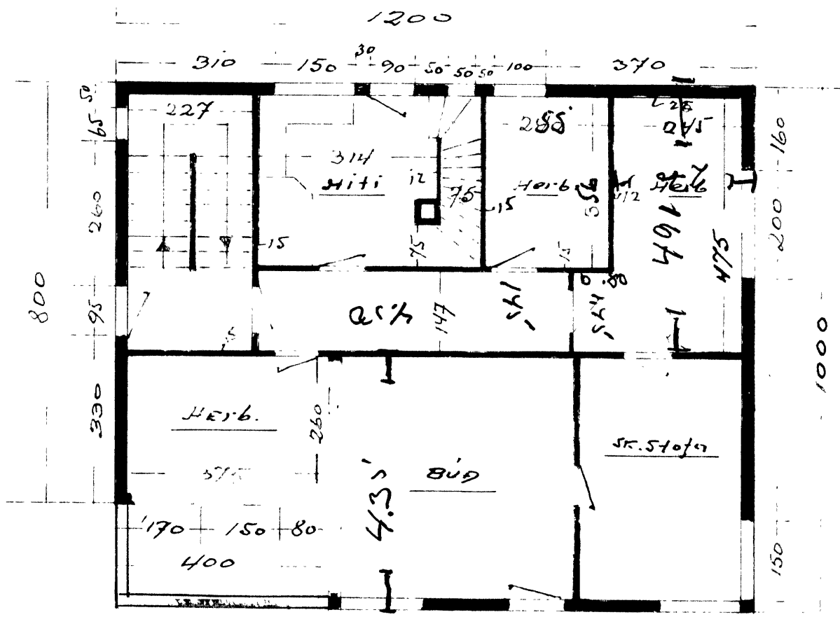
1. HÆÐ 12.12
