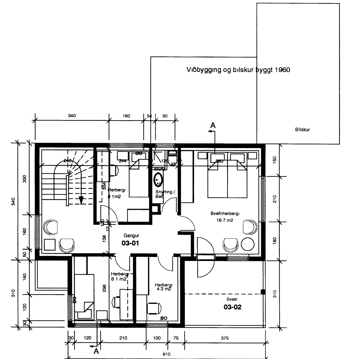
Grunnmynd 3 hæðar
