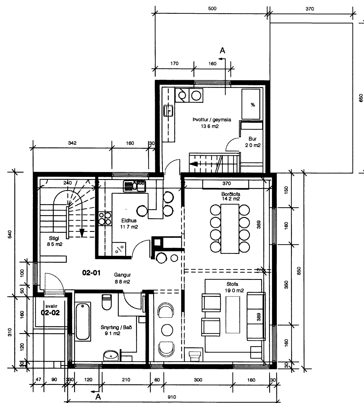
Grunnmynd 2 hæðar
