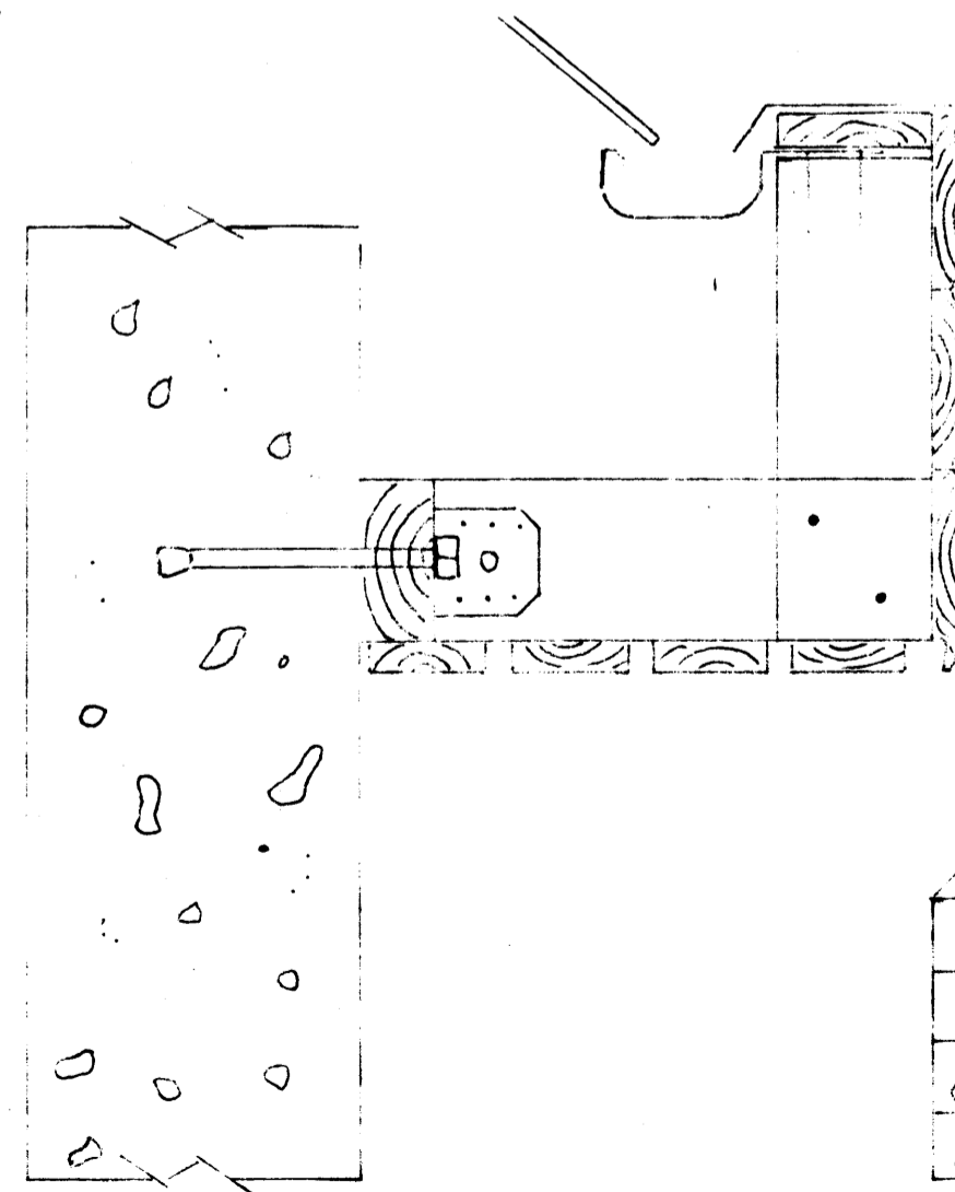
Þakkantur 1:20
