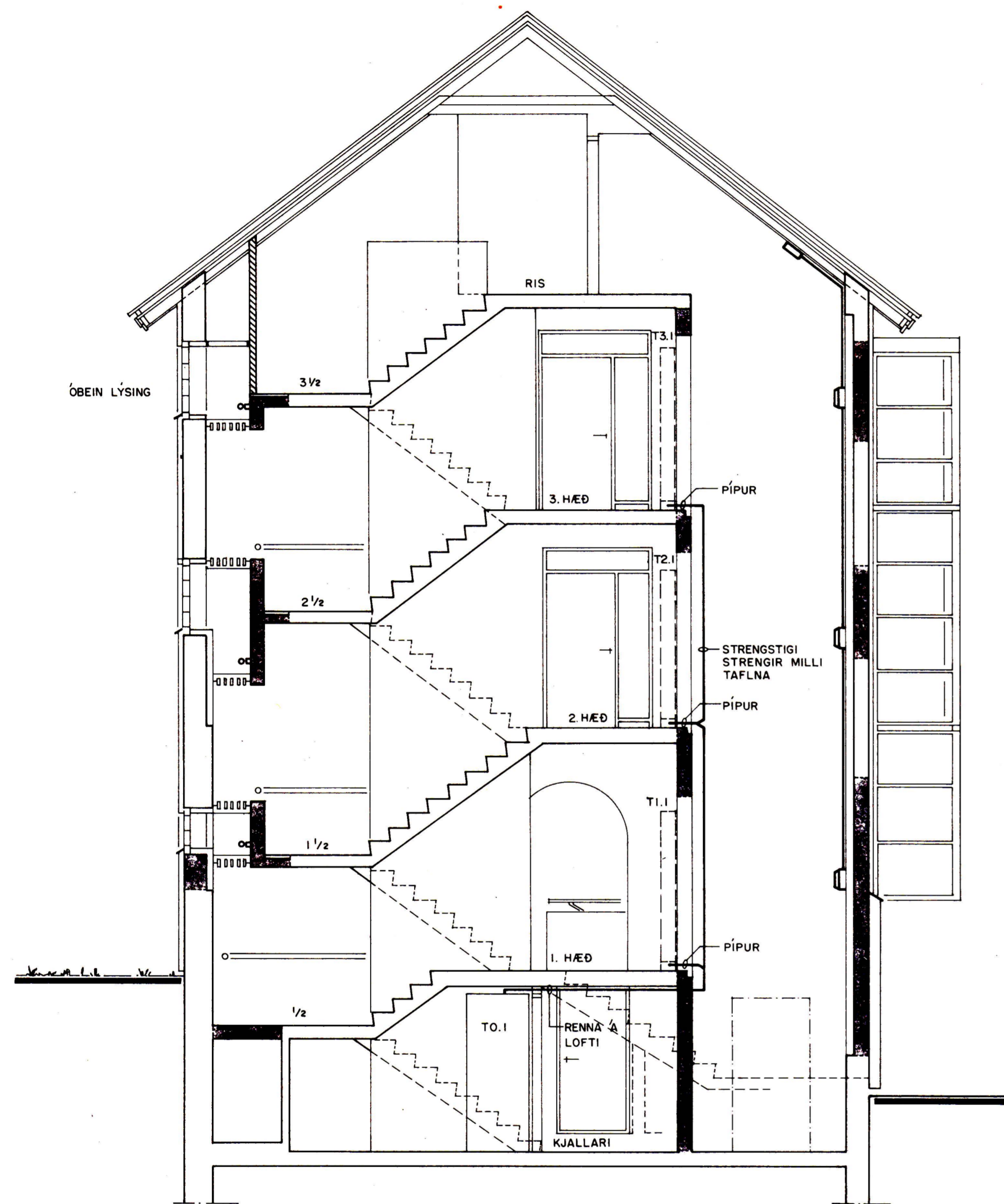
SNEIÐING M. 1:50
