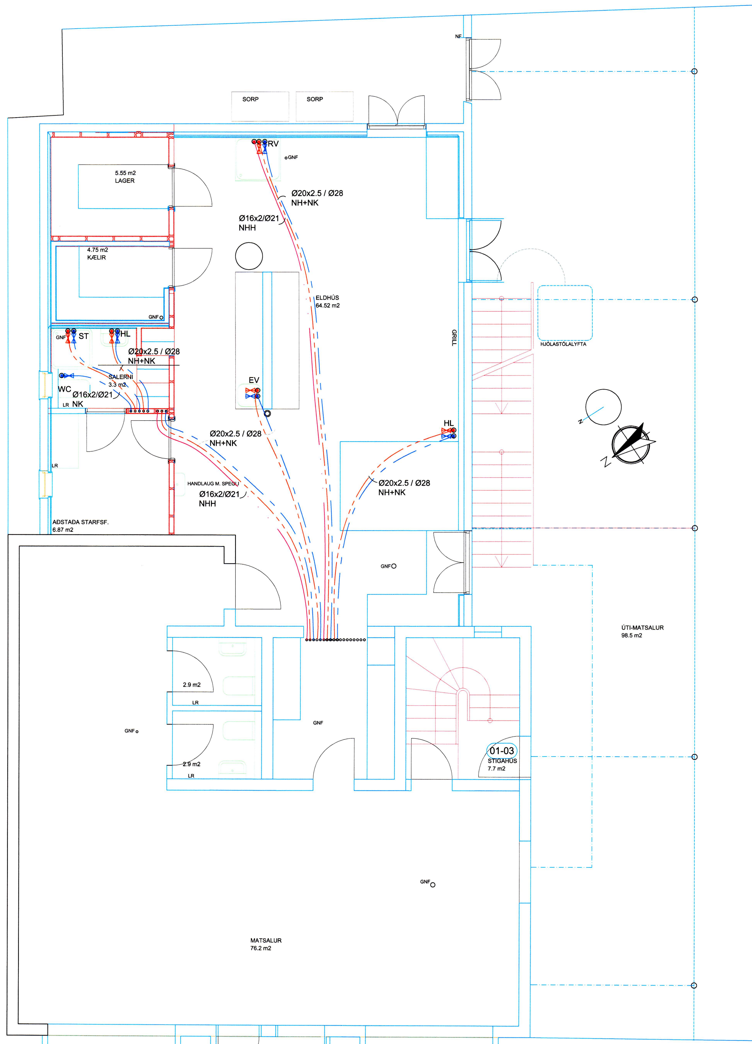
NEYSLUVATNSLAGNIR
