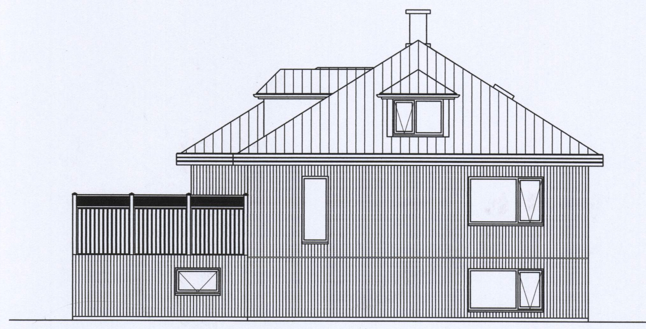
SUÐURHLIÐ M=1:100
