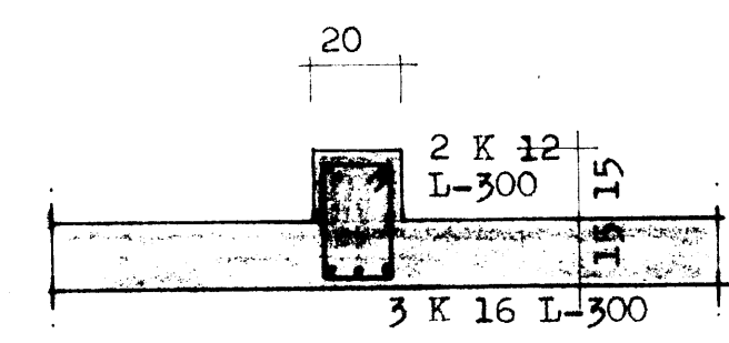
SNID - B 1:20
