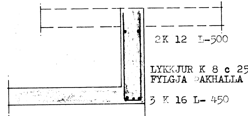
SNID - A 1:20 I PLOTU VID ÚTVEGG
