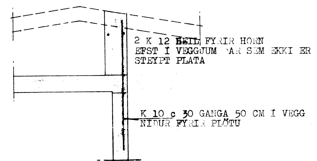
SNID - E 1:20
