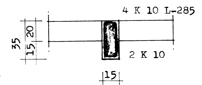
SÖLA S-2 1:20
