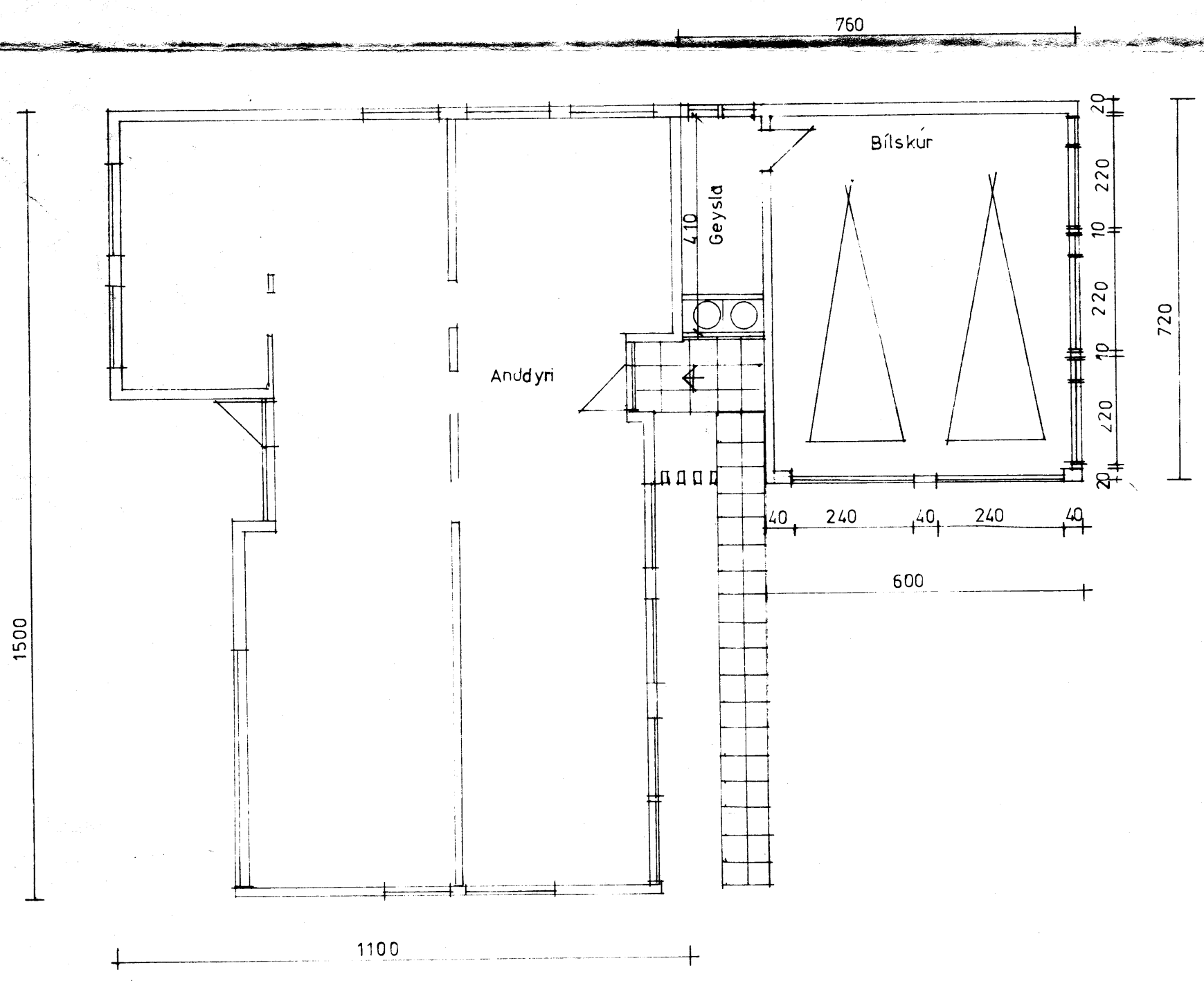
GRUNNMYND
