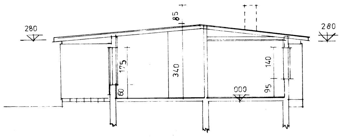
SNEIDING A-A
