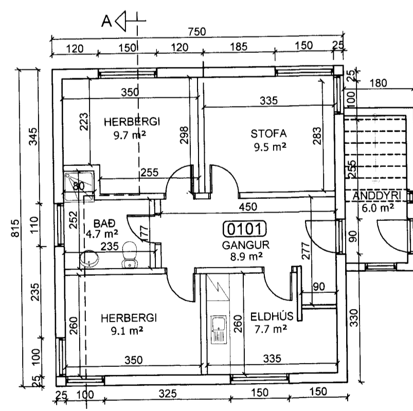
GRUNNMYND 1.HÆÐ
