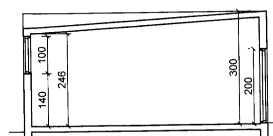
SNÍÐ B-B
