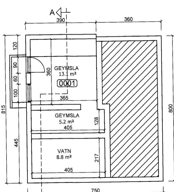
GRUNNMYND KJALLARI
