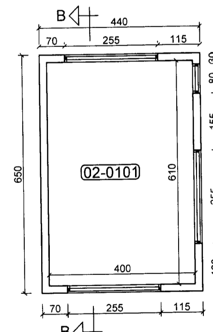
GRUNNMYND BÍLSKUR
