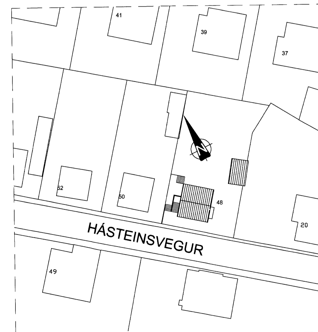
AFSTÖÐUMYND M : 1.500
