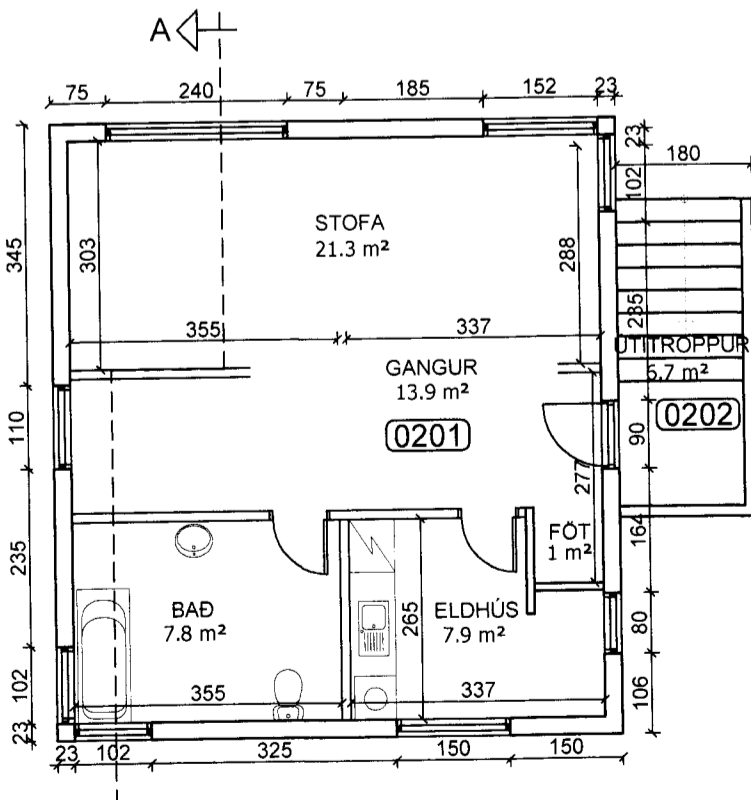
GRUNNMYND 2.HÆÐ
