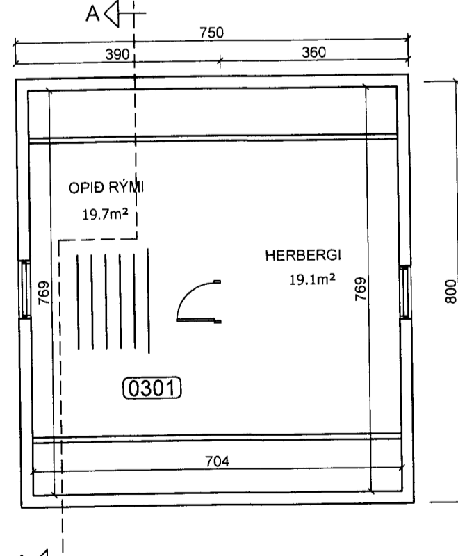
GRUNNMYND RIS
