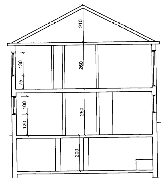
SNÍÐ A-A
