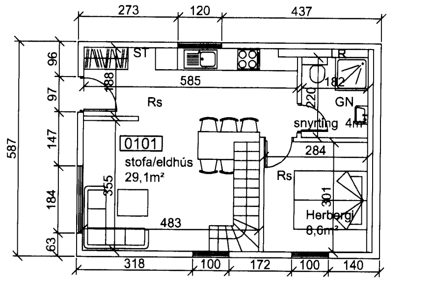
grunnmynd neðri hæð mkv 1:100
