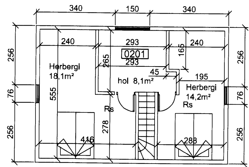
grunnmynd efri hæð mkv 1:100
