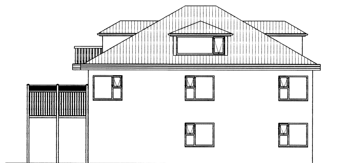
AUSTURHLIÐ M=1:100
