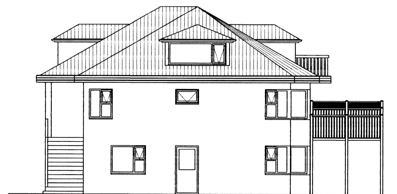
VESTURHLIÐ M=1:100
