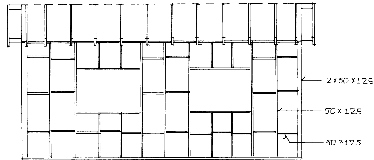
AUSTURHLIÐ M=1:50
