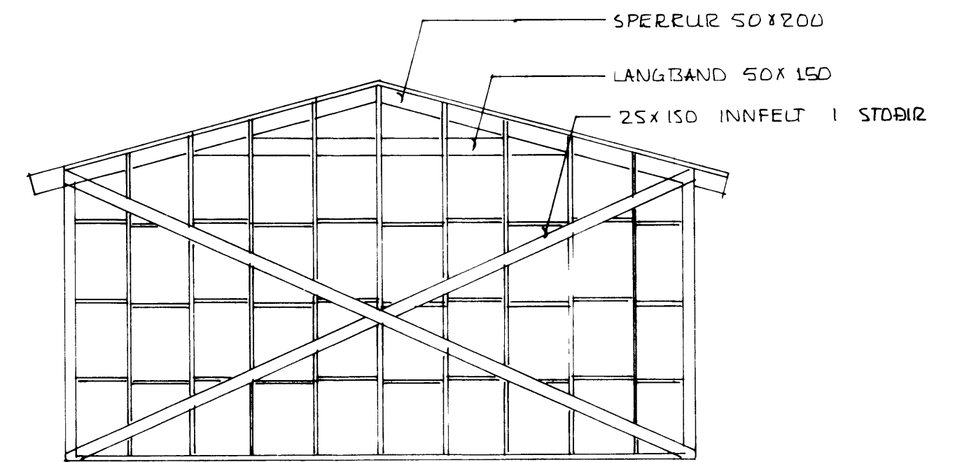
NORÐURHLIÐ M=1:50
