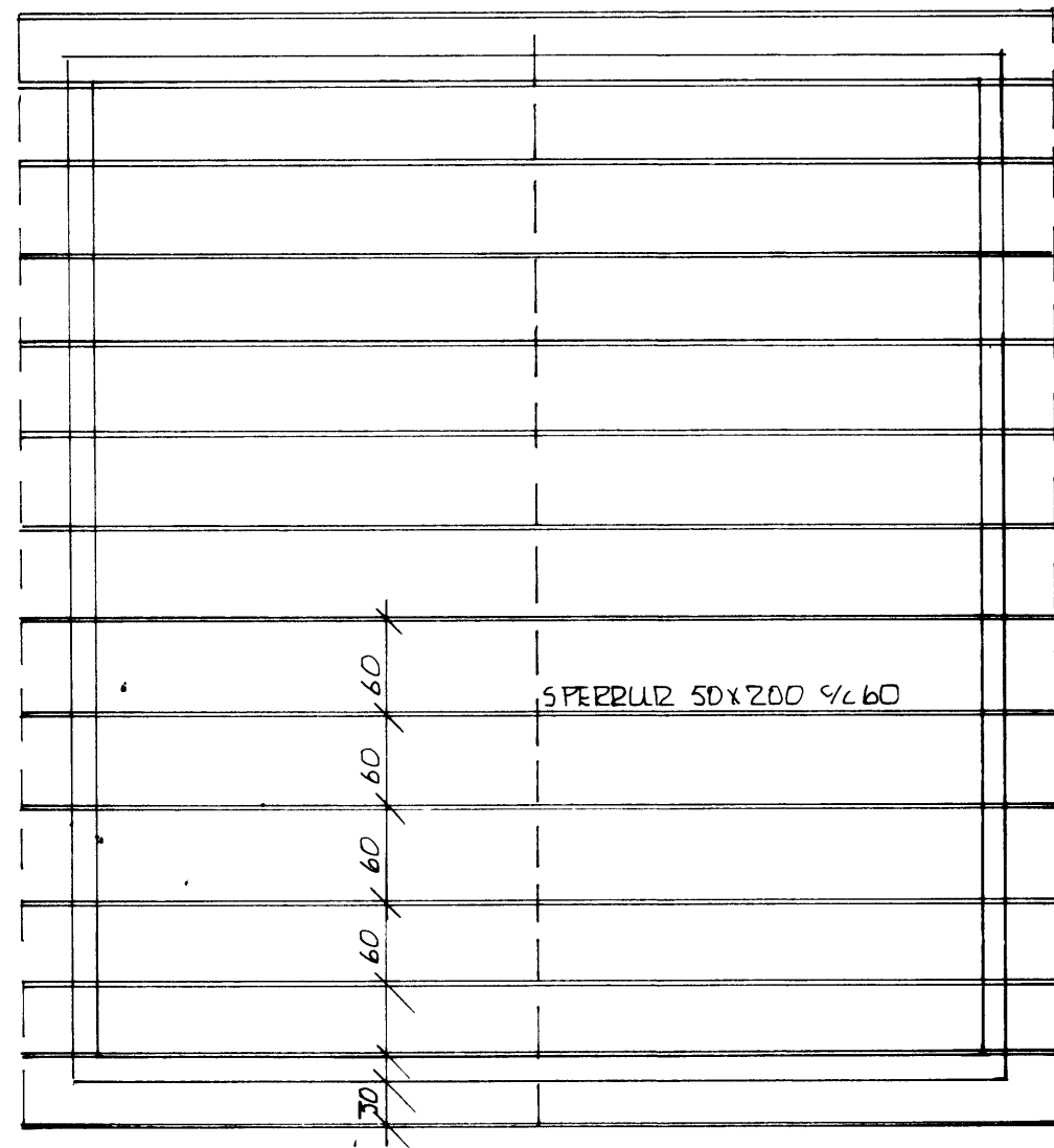
GRUNNMYND ÞAKVIRKI M=1:50
