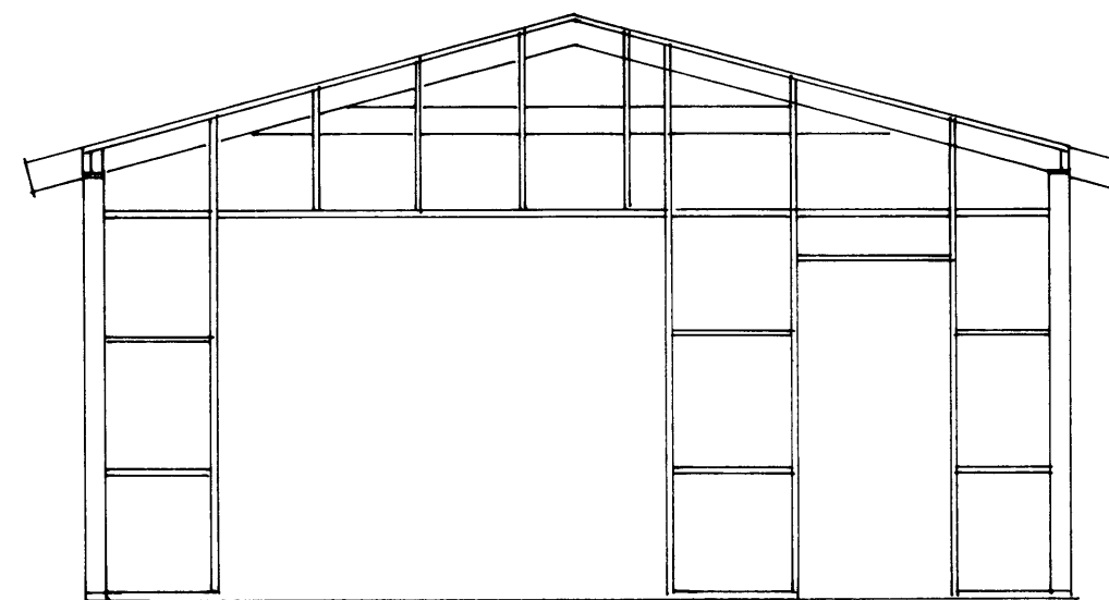
SUÐURHLIÐ M=1:50
