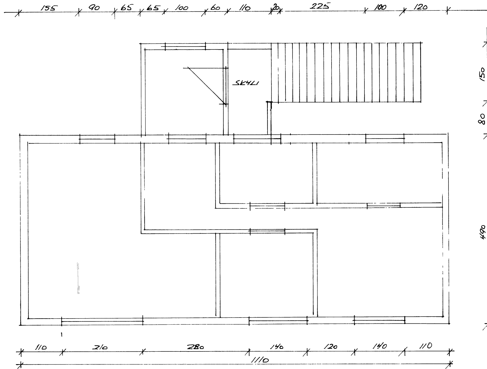
GRUNNMYND 2 HÆÐ
