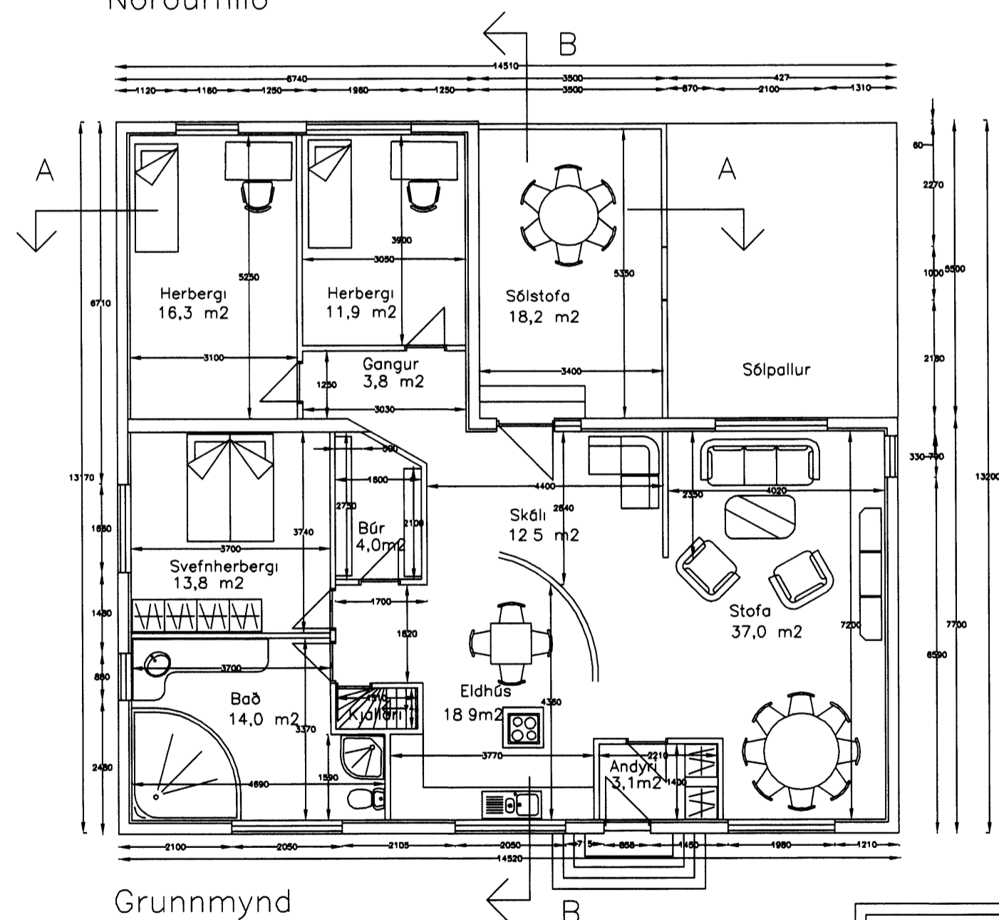
Norðurhlíð
