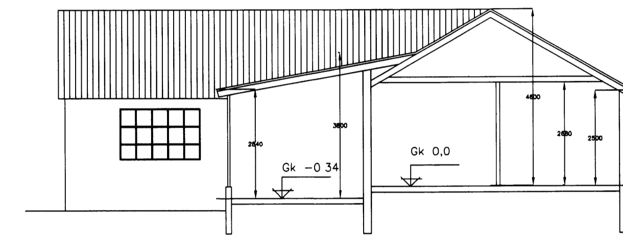
Snið A-A
