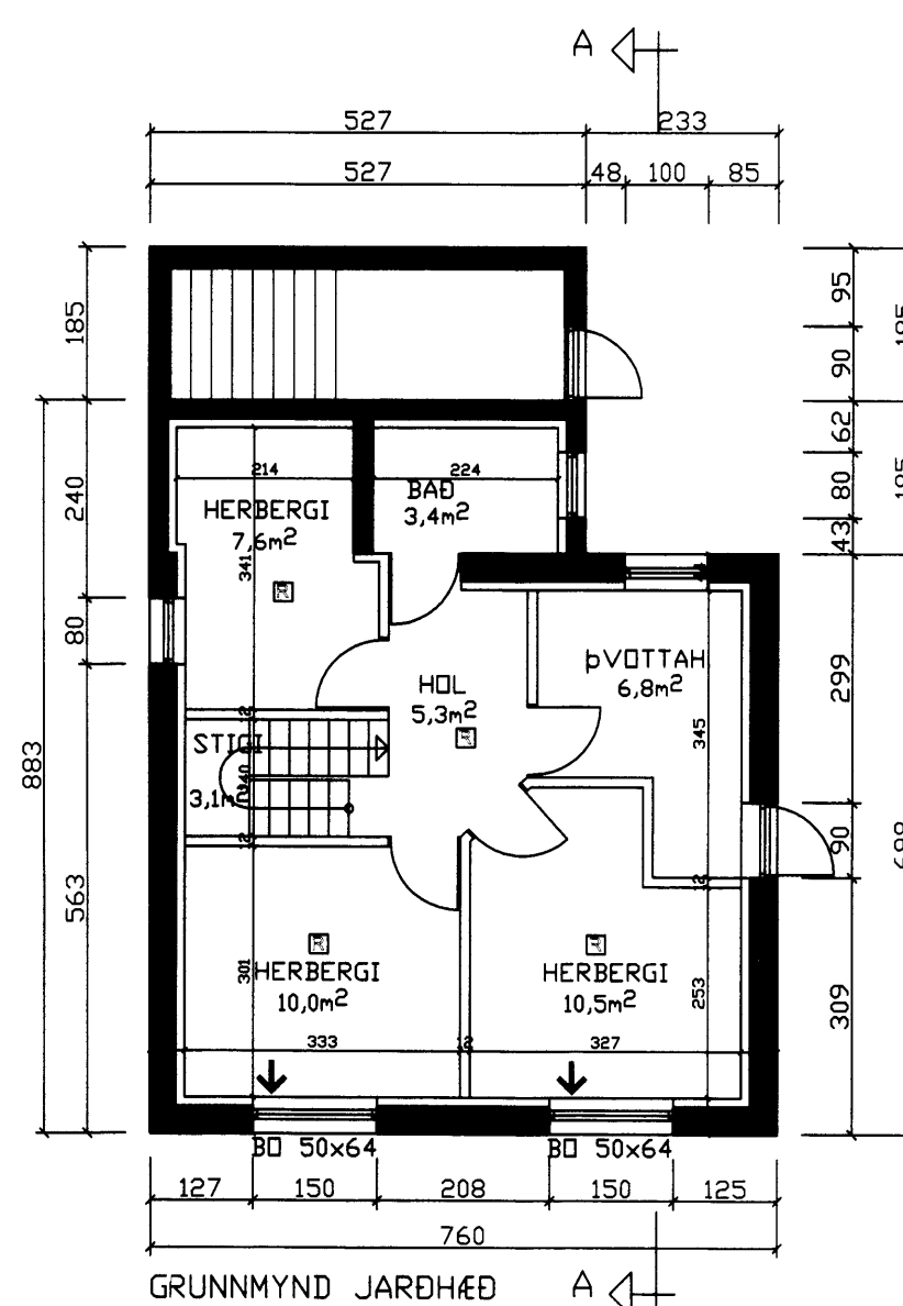
GRUNNMYND JARDHED
