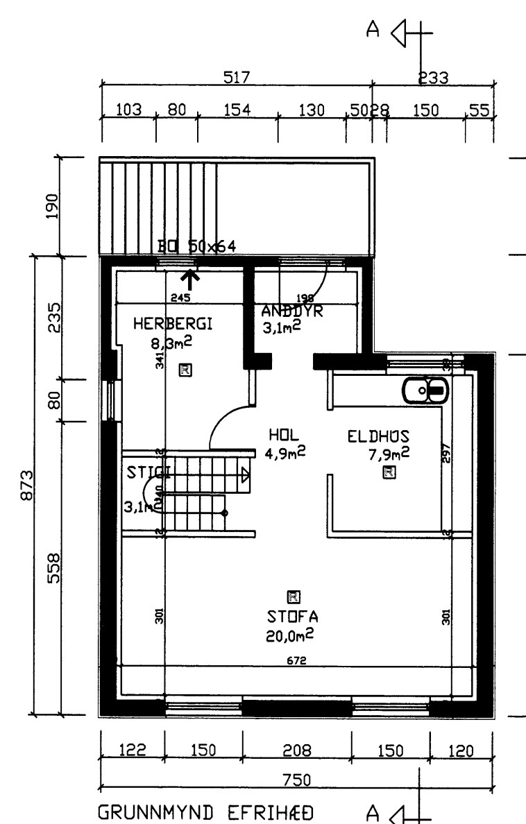
GRUNNMYND EFRIHED
