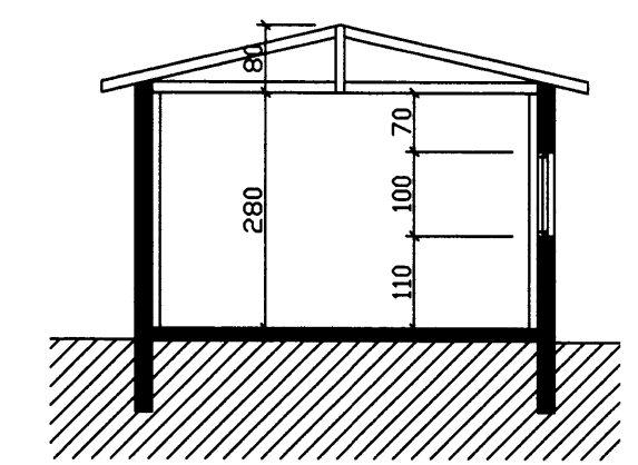
SNID B-B M=1:100
