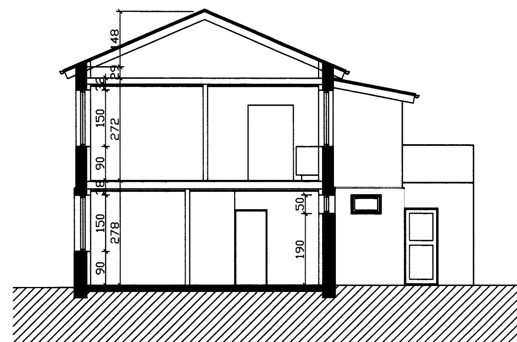
SNID A-A M=1:100
