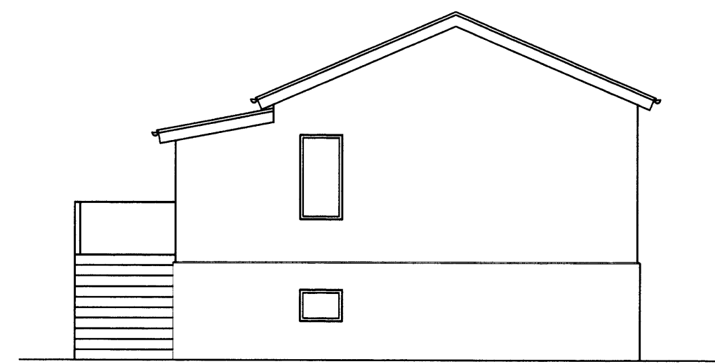
VESTURHLID M=1:100
