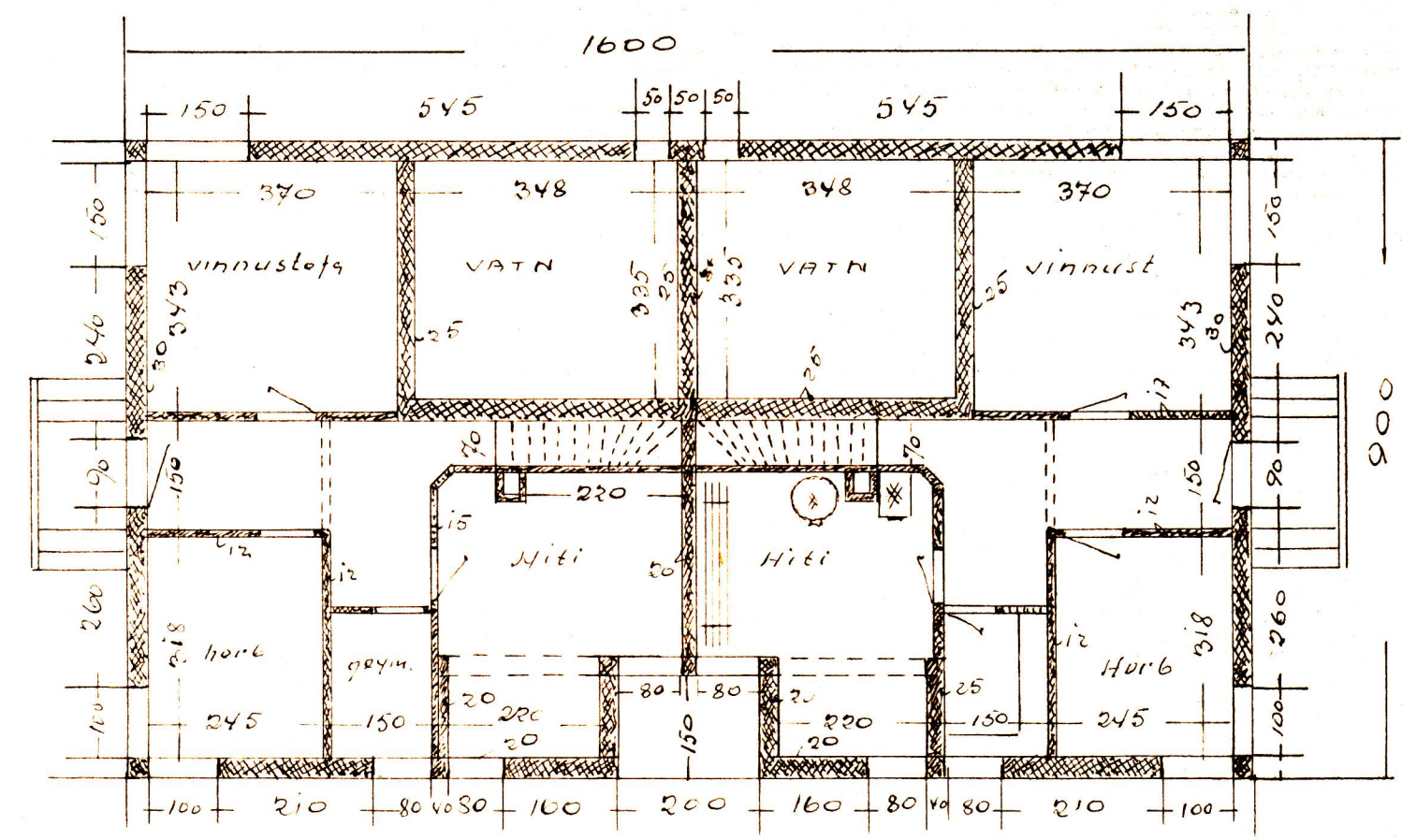
Kjallari
