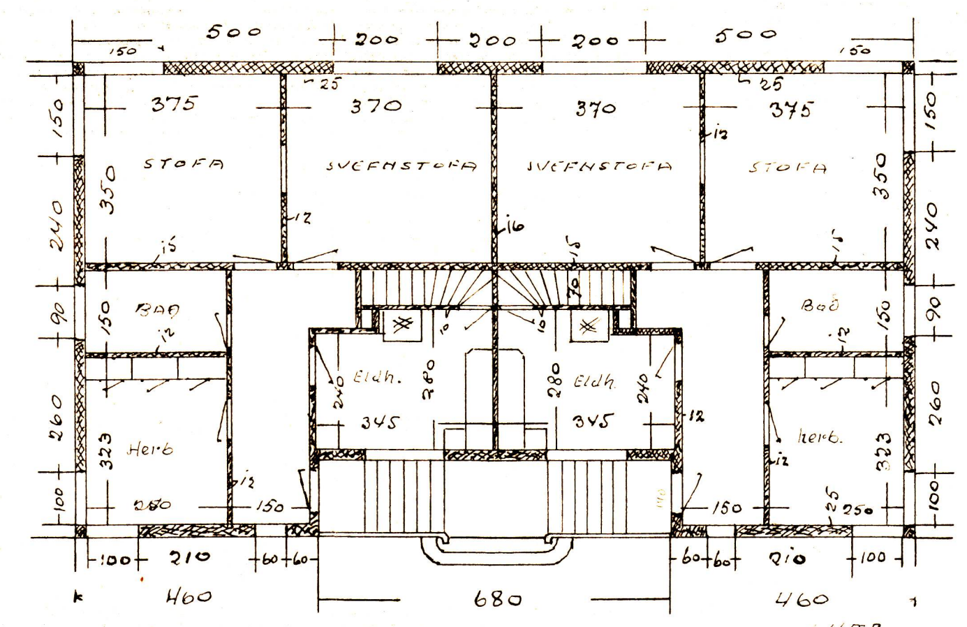
1. HÆÐ
