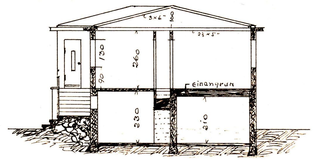
SKURÐUR
