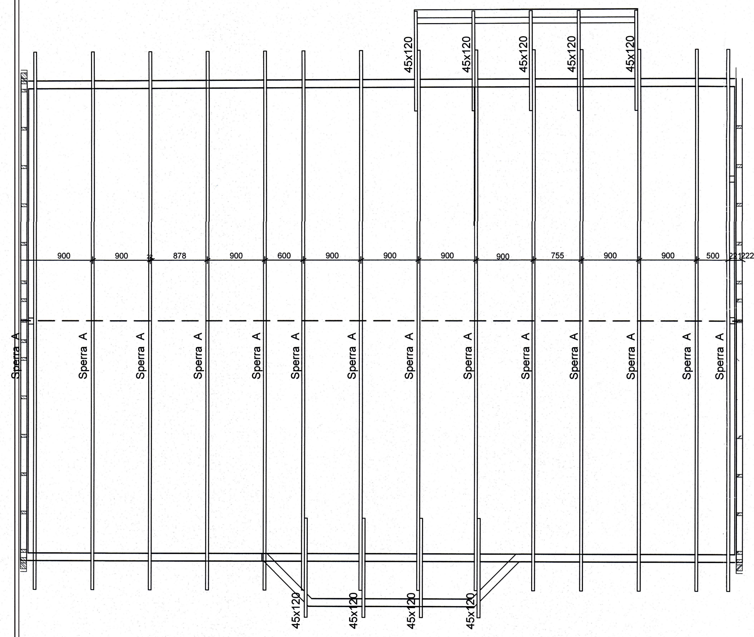
Grunnmynd Mkv. 1:50
