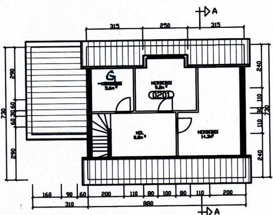
GRUNNMYND RIS M=1:100
