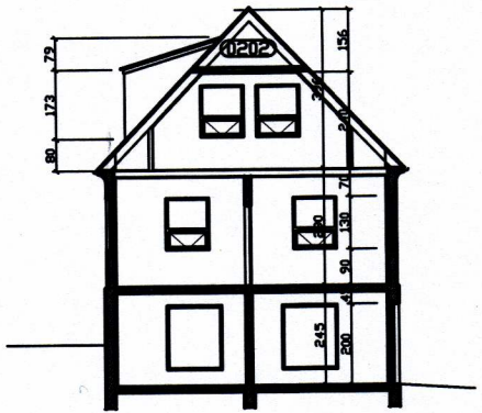
SNID A-A M=1:100
