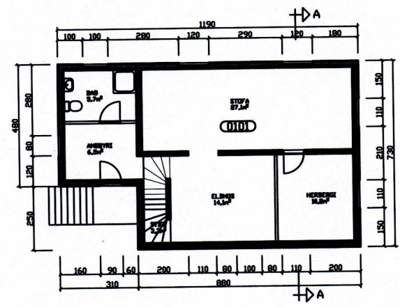
GRUNNMYND 1. HÆÐ M=1:100
