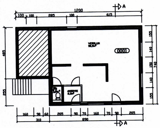
GRUNNMYND KJALLARI M=1:100
