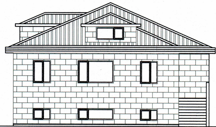
NORDURHLID
