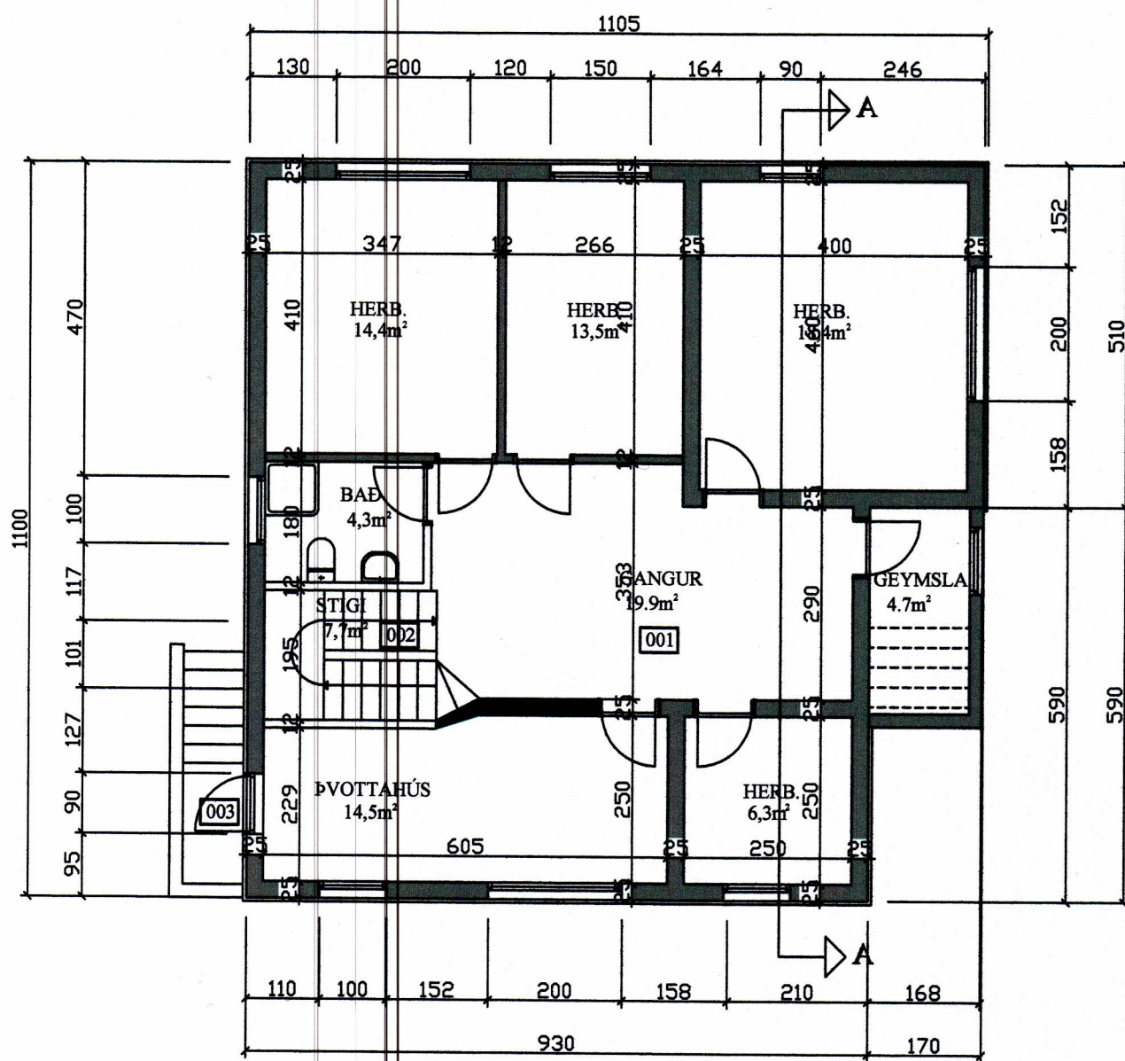
GRUNNMYND KJALLARI
