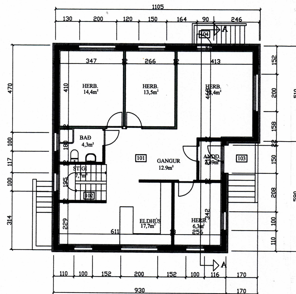
GRUNNMYND 1. HÆÐ
