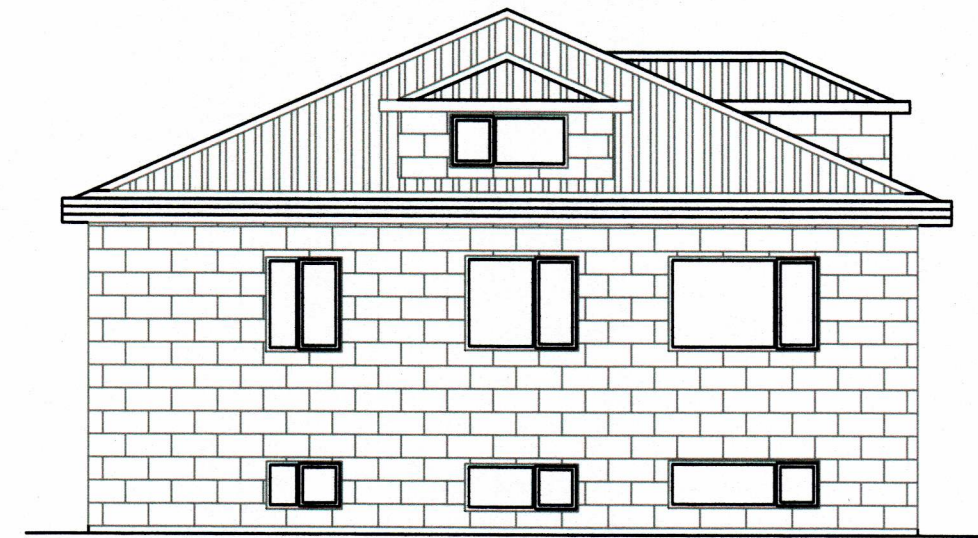
SUDURHLID
