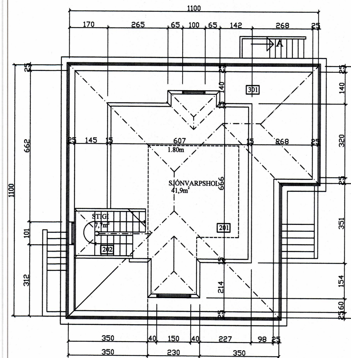
GRUNNMYND 2. HÆÐ
