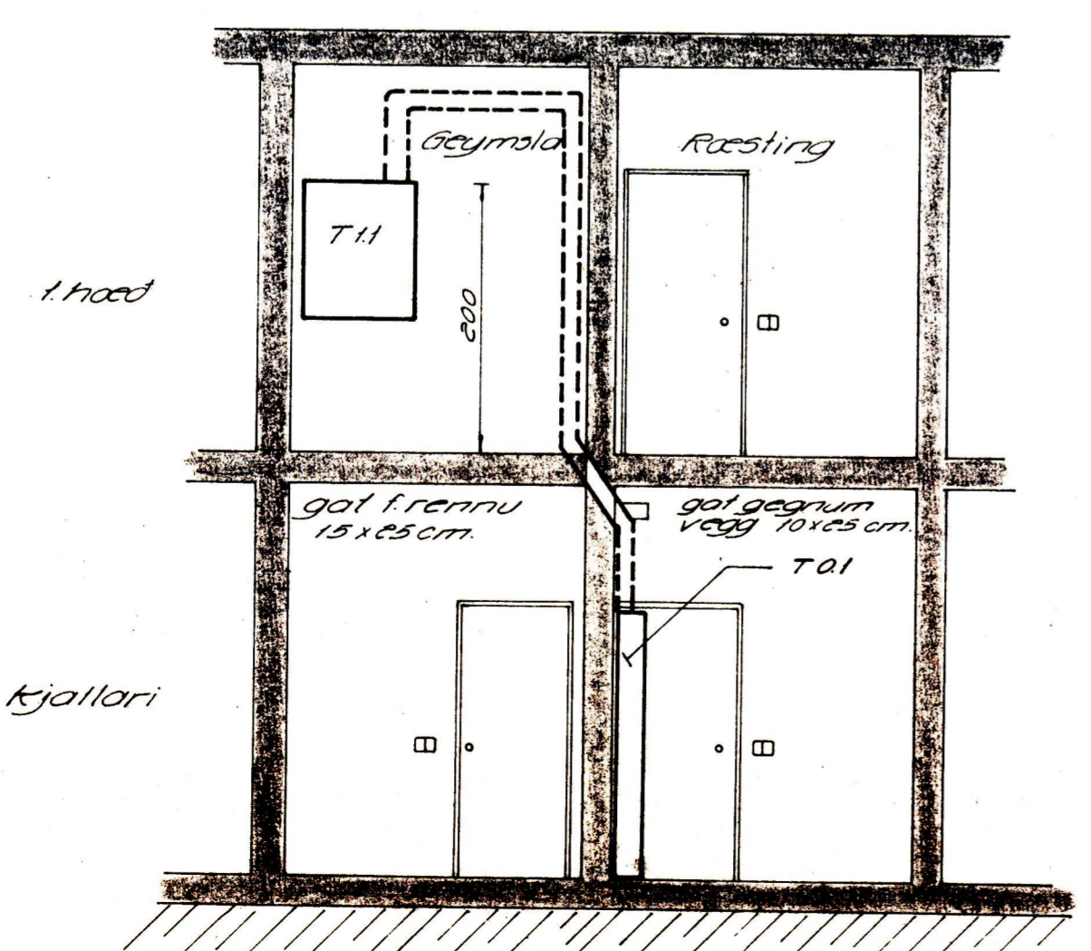
Snid A-A
