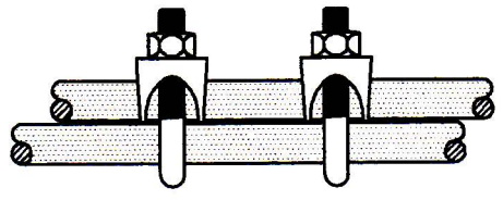
FRÁGANGUR Á SAMTENINGUM STEYPUVEINA FYRIR SÖKKULJARÐSKAUT
