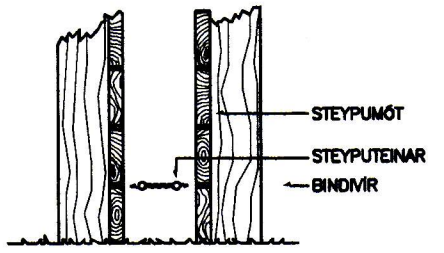
SNID Í STEYPUMÓT
