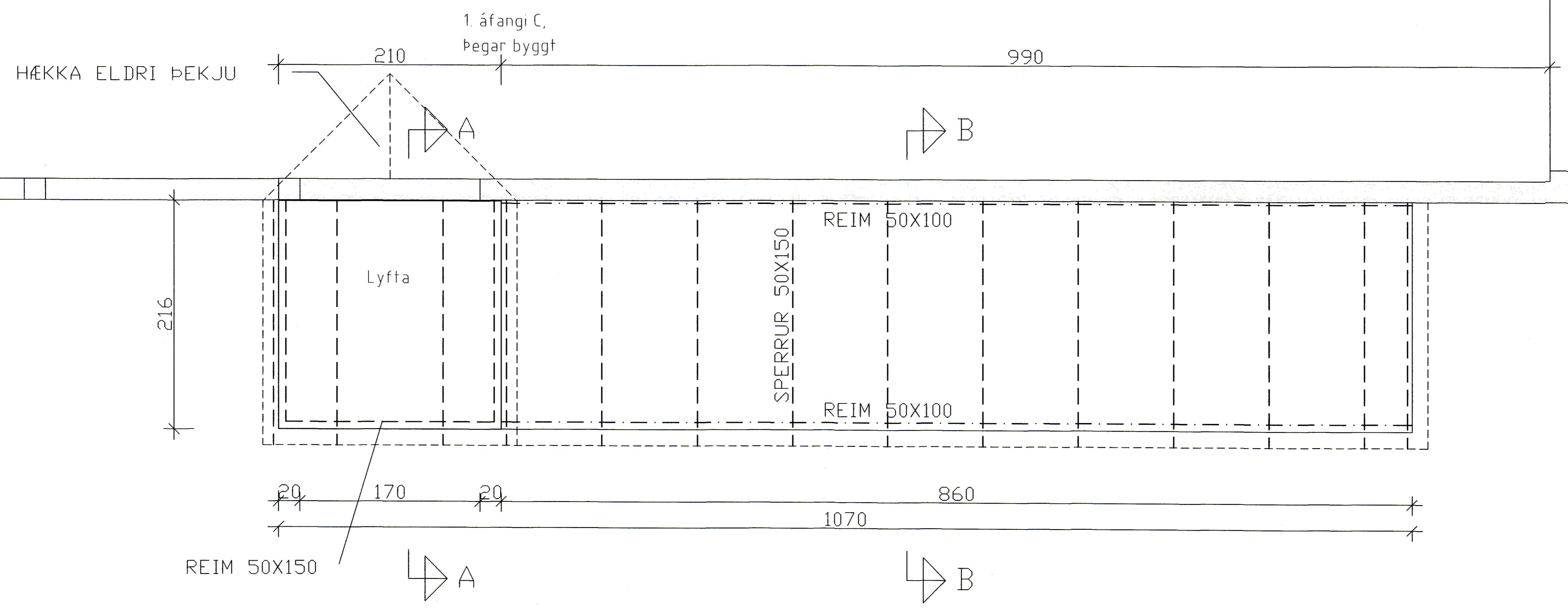
GRUNNMYND ÞAKSPERRUR
