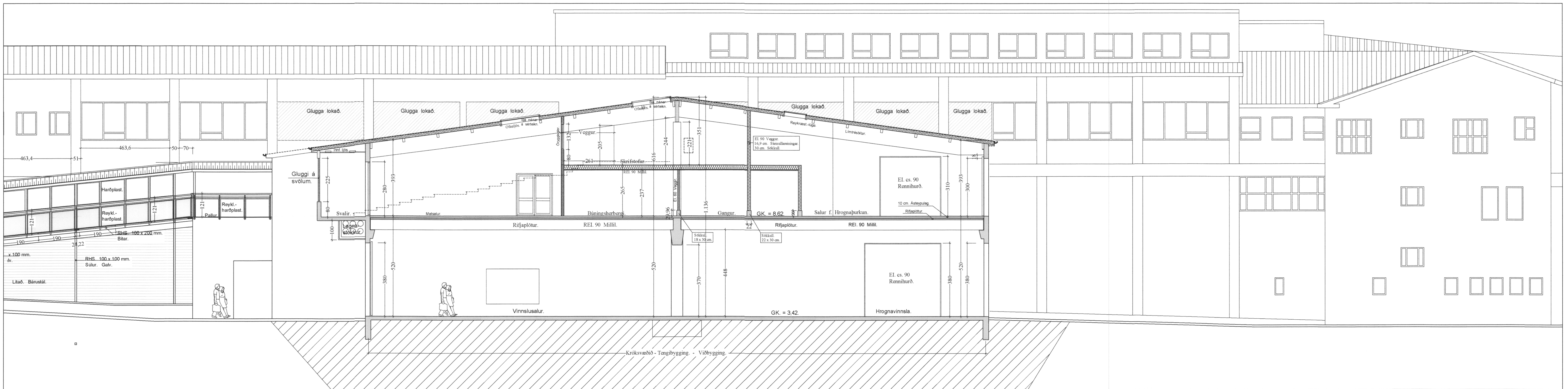
Sneiðing E-E í Tengibygggingu -- Austurhlíð. 1:100
