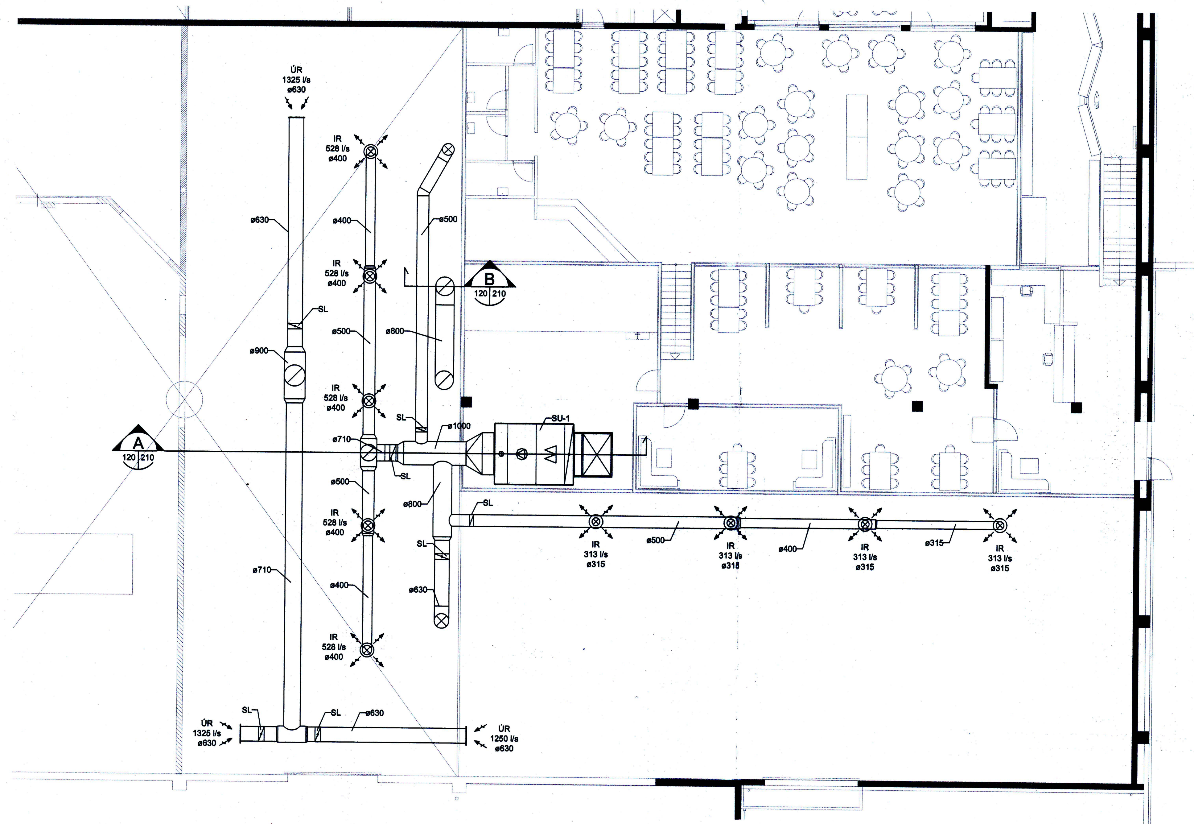
GRUNNMYND 3. HÆÐ 1:100
