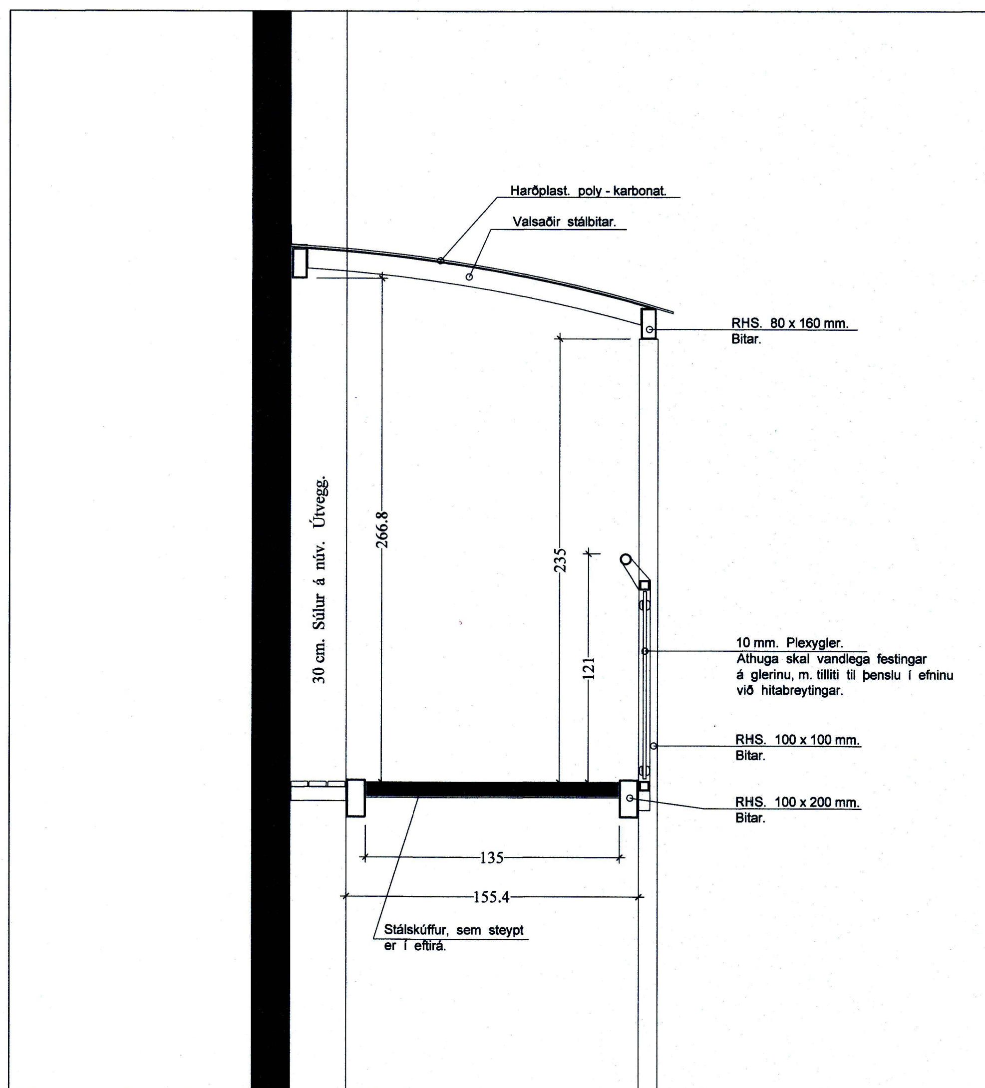
Sneiðing. Hlutamynd. 1:20
