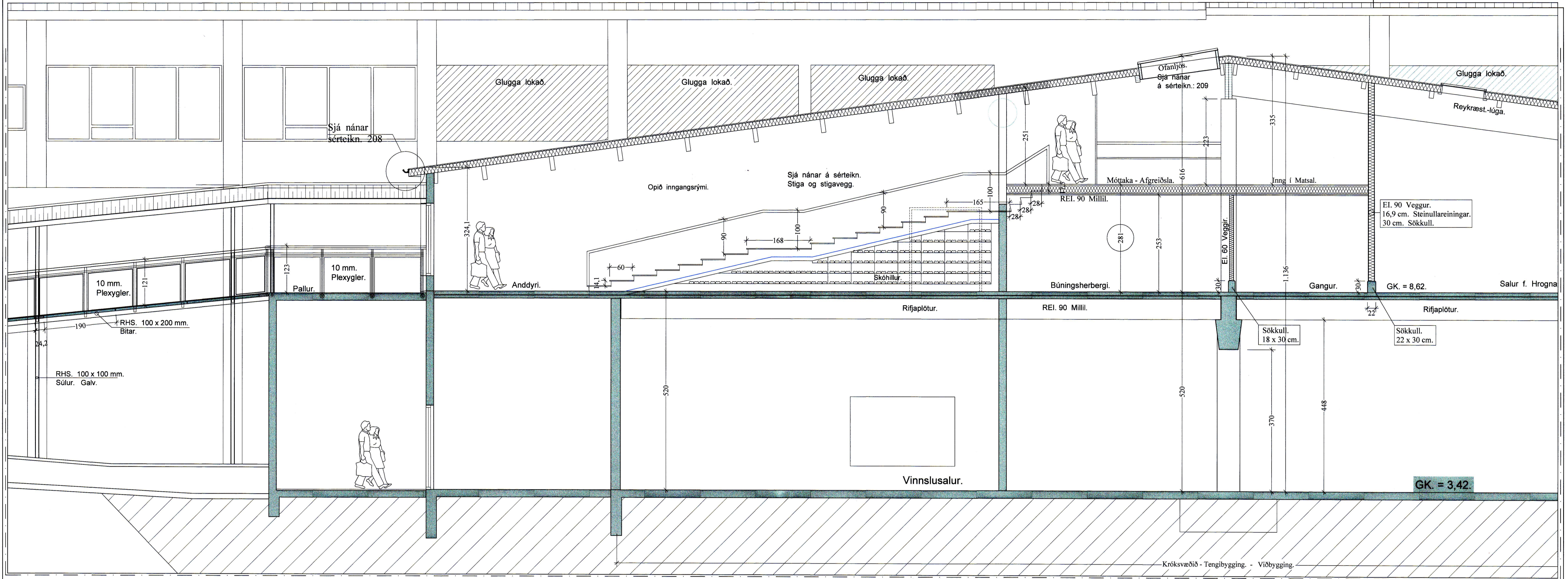
Sneiðing F-F í Tengibyggingu -- Gegnum Aðalinnang. Vesturhlíð. 1:50
