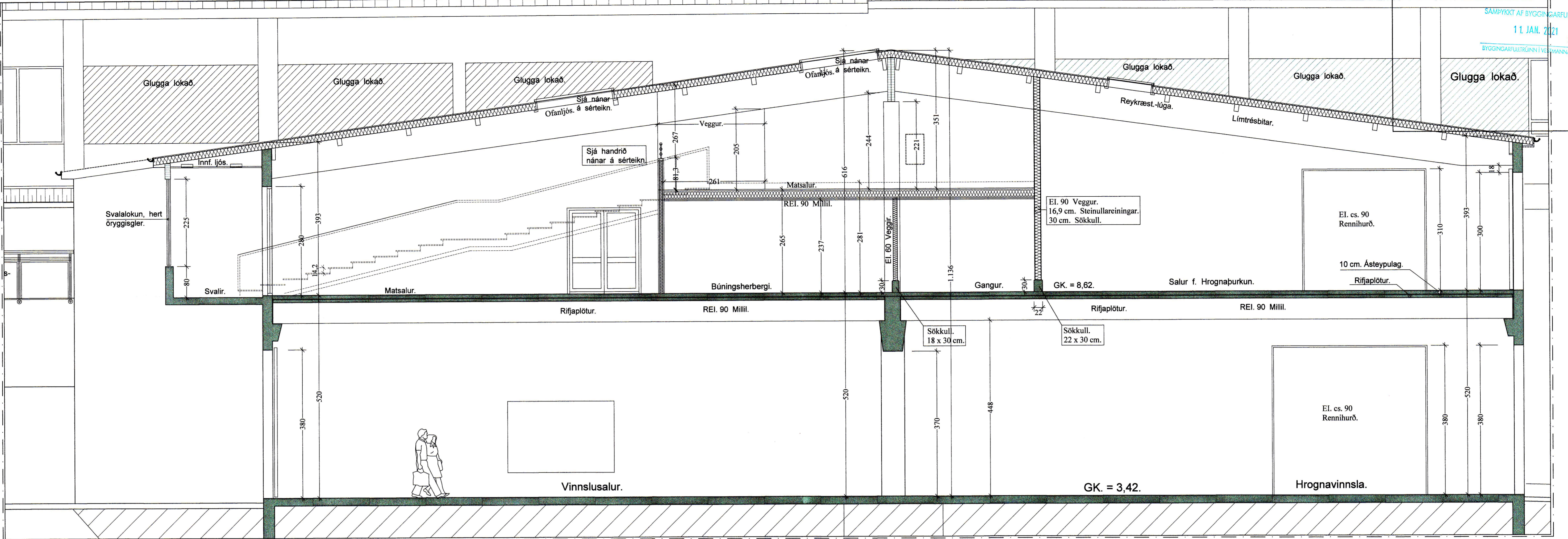
Sneiðing E - E í Tengibyggingu -- Vesturhlíð. 1:50
