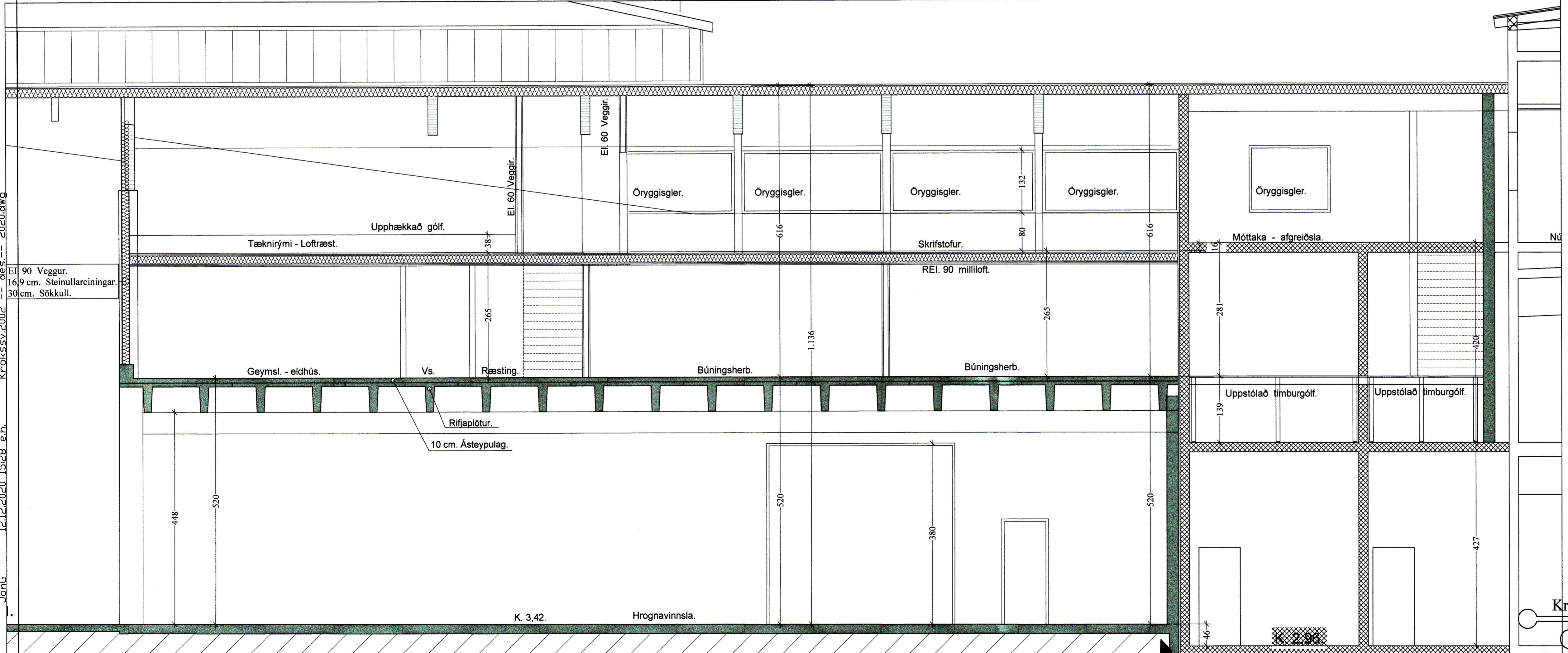
Sneiðing í viðbyggingu yfir Hfnargötu. B - B 1:50
