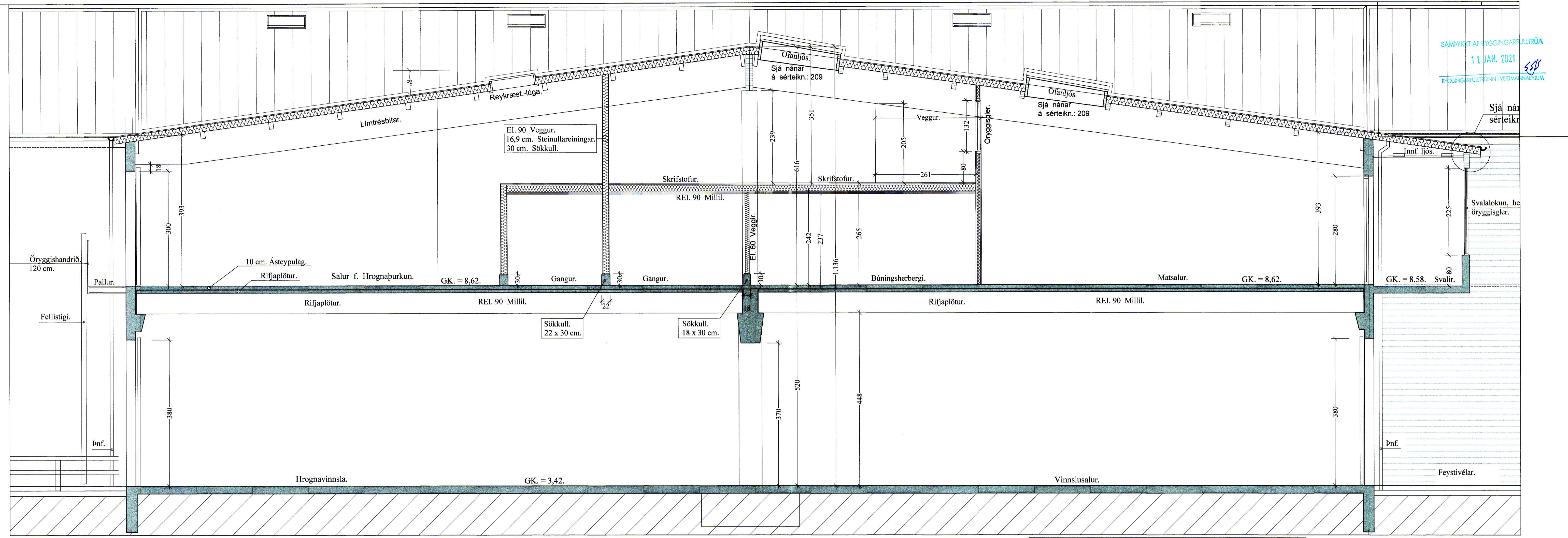
Sneiðing D-D í Tengibyggingu -- Vesturhlíð. 1:50
